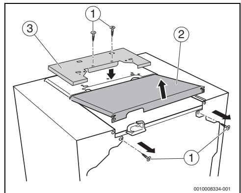
Bild 7 Hintere Kesselhaube abnehmen/Adapterblech montieren
