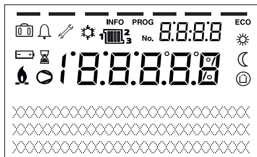
Abb.4 Symbole im Display
