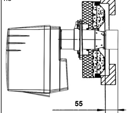
Montaggio tubo ausiliario
