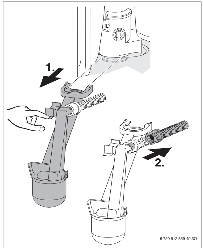
Bild 44 Kondensatsiphon
