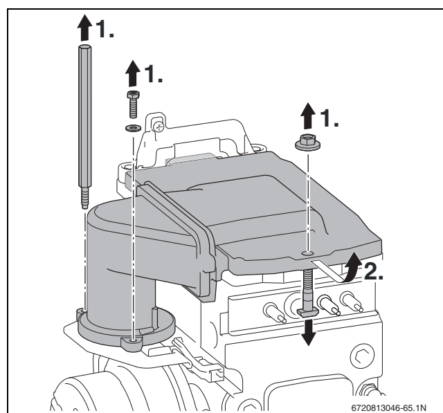
Bild 41 Brennerdeckel ausbauen
