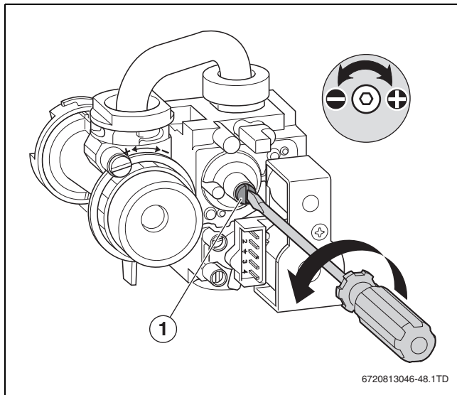
Bild 30 Schraube entfernen
