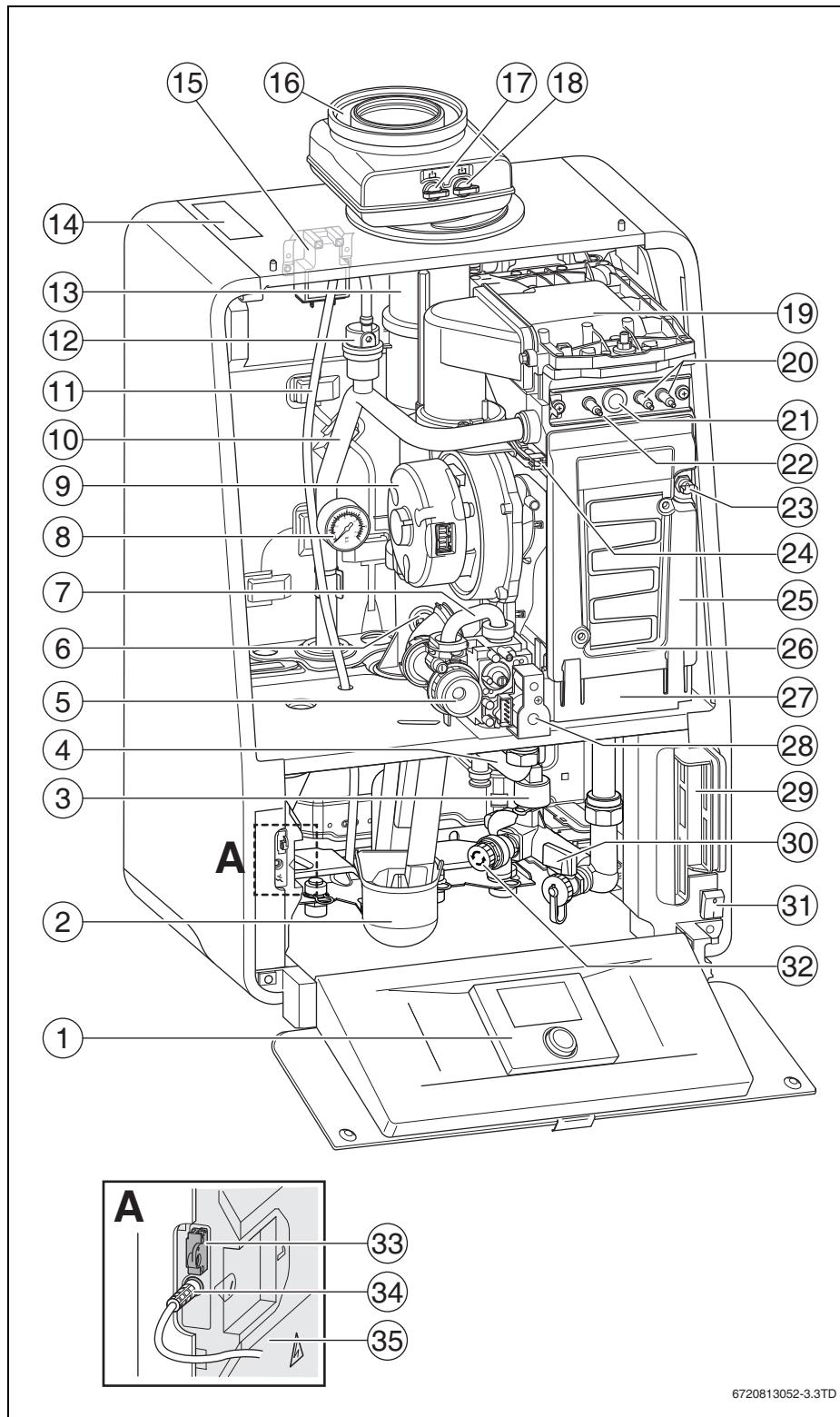
Bild 3 GC9000iW 20/30/40/50 H
