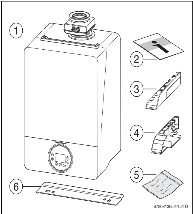
Bild 1 GC9000iW 20/30/40/50 H oder GC9000iW 20/30 E(B)
