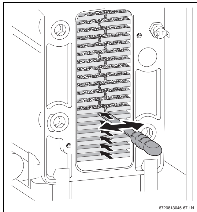
Bild 46 Reinigungsmesser
