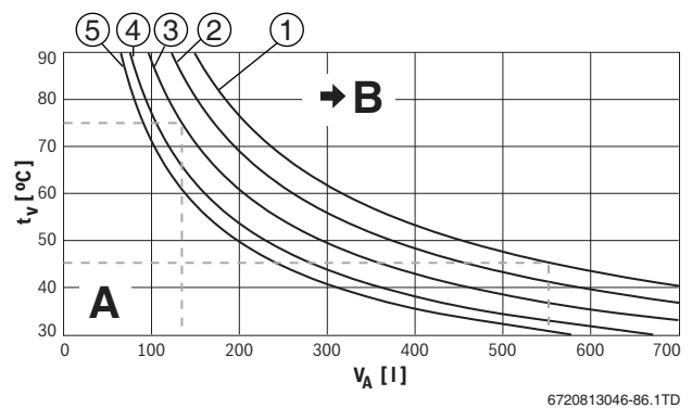
Bild 18 Kennlinien des Ausdehnungsgefäßes, Heizungsausdehnungsgefäß 14 l
