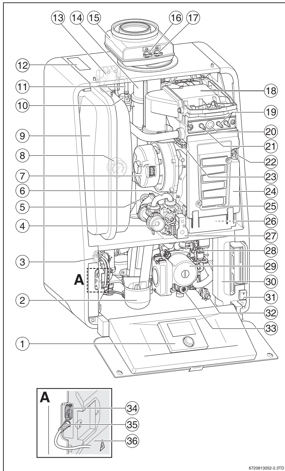
Bild 2 GC9000iW 20/30 E(B)
