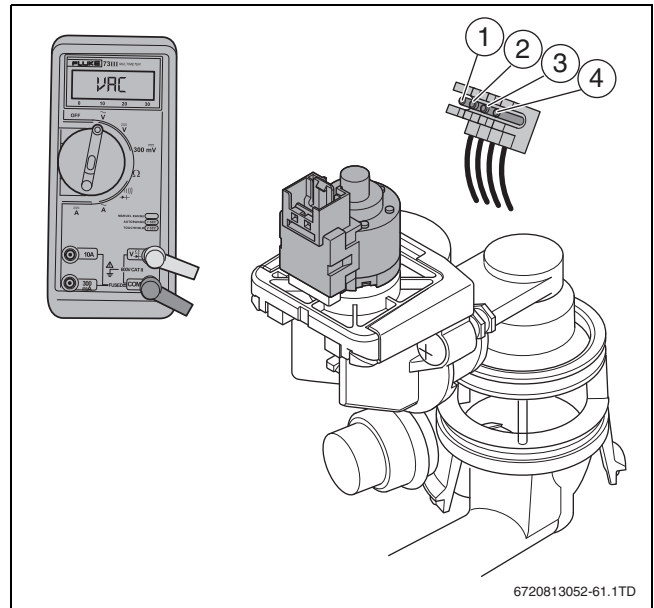
Bild 50 3-Wege-Ventil
