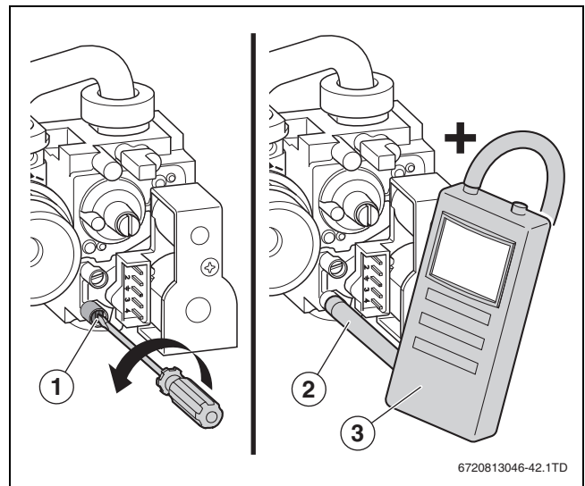
Bild 27 Gas-Anschlussdruck messen
