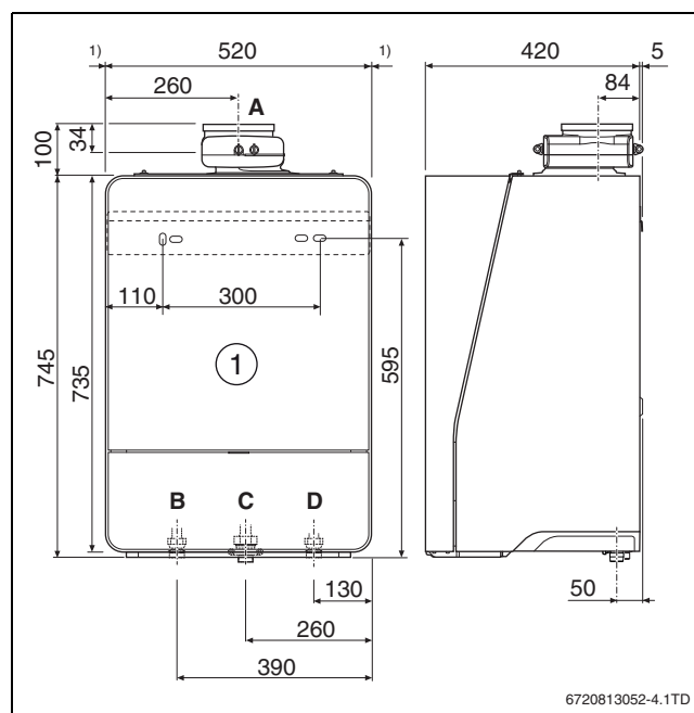
Bild 5 Typ H - Abmessungen und Anschlüsse [mm] 1) Servicemaßen, im Schrank eingebaut, können 0 mm sein.
