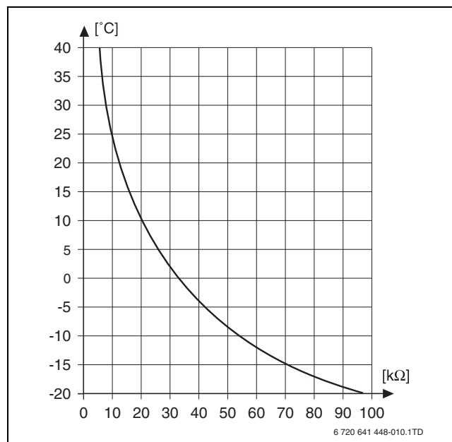
Bild 10 Widerstandskennlinie für Außentemperaturfühler
