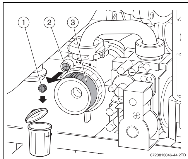
Bild 28 Plombe entfernen
