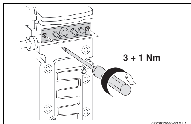
Bild 39 Elektroden-Set montieren
