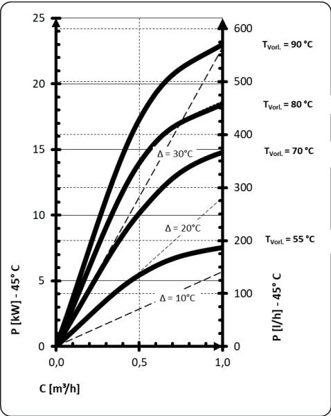
SPEICHER-LEISTUNGSDIAGRAMM
