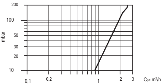
DRUCKVERLUST HEIZUNGSSEITE
