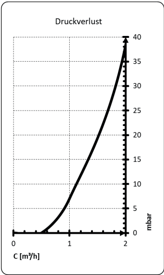
DRUCKVERLUST HEIZUNGSSEITE
