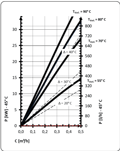
SPEICHER-LEISTUNGSDIAGRAMM
