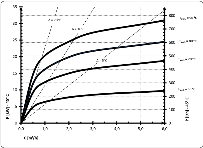
SPEICHER-LEISTUNGSDIAGRAMM
