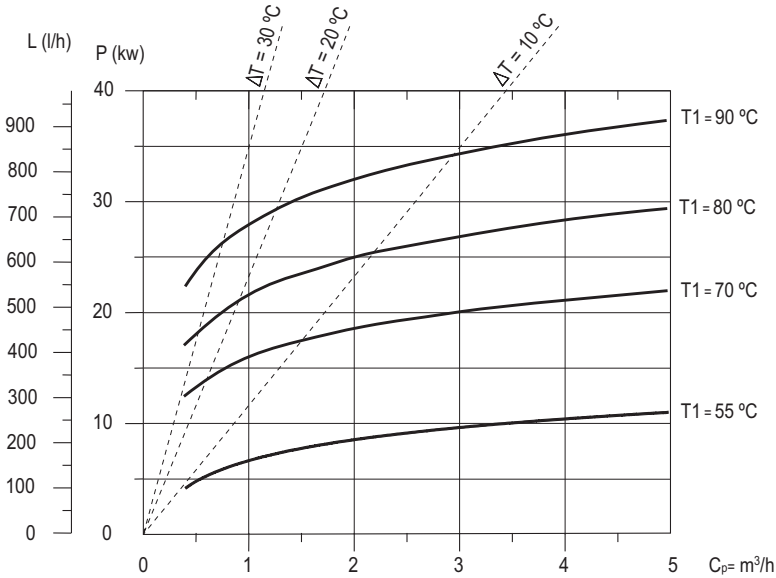
SPEICHER-LEISTUNGSDIAGRAMM
