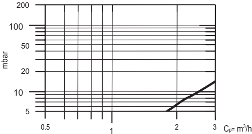
DRUCKVERLUST HEIZUNGSSEITE
