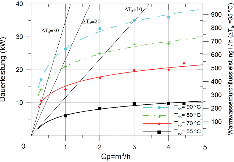
SPEICHER-LEISTUNGSDIAGRAMM
