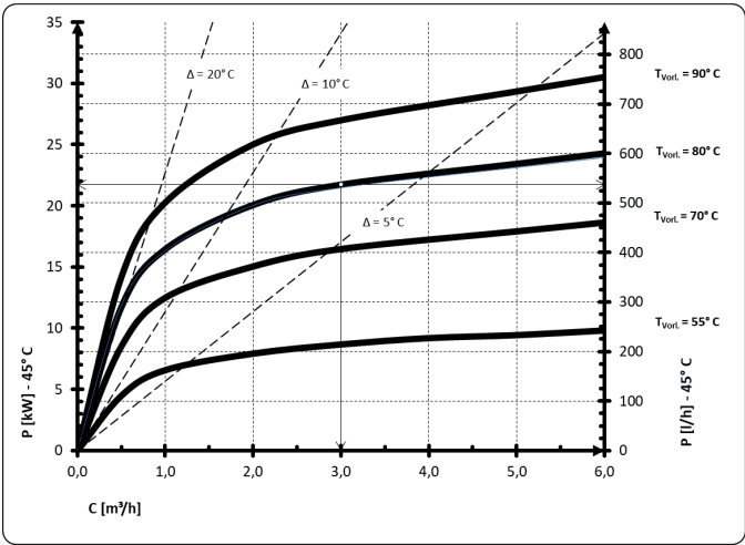
SPEICHER-LEISTUNGSDIAGRAMM
