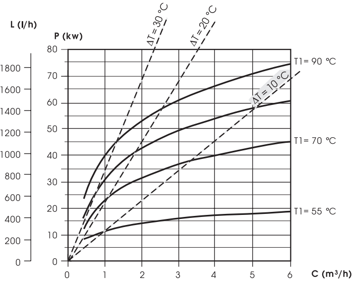
SPEICHER-LEISTUNGSDIAGRAMM
