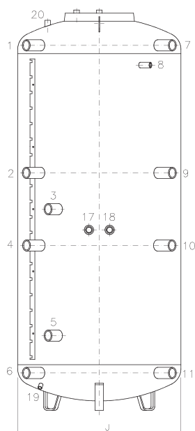
Vorderansicht
