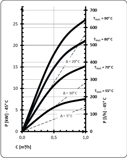
SPEICHER-LEISTUNGSDIAGRAMM
