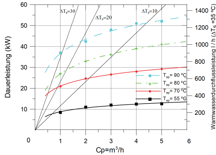
SPEICHER-LEISTUNGSDIAGRAMM
