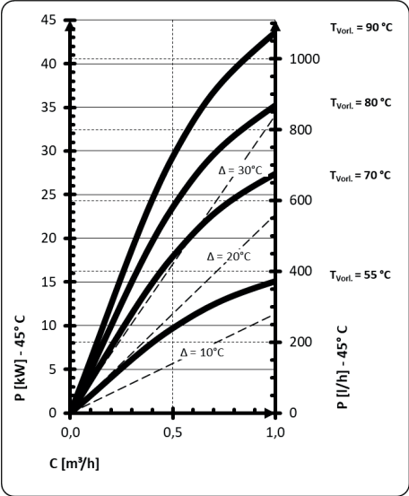
SPEICHER-LEISTUNGSDIAGRAMM
