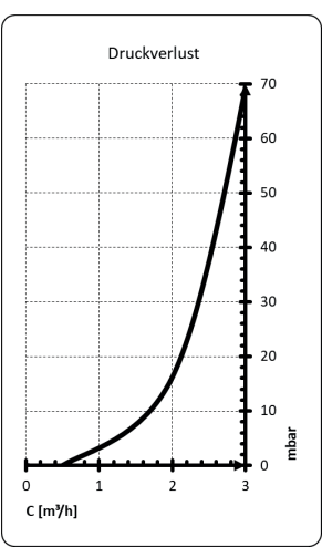
DRUCKVERLUST HEIZUNGSSEITE
