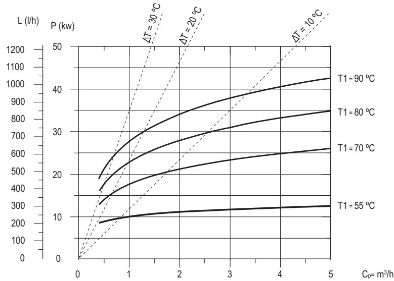
SPEICHER-LEISTUNGSDIAGRAMM
