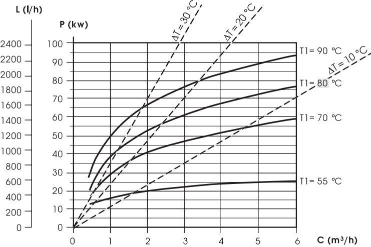
SPEICHER-LEISTUNGSDIAGRAMM
