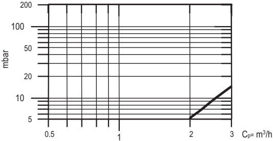
DRUCKVERLUST HEIZUNGSSEITE
