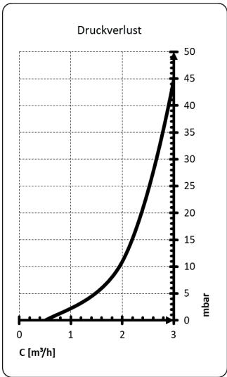
DRUCKVERLUST HEIZUNGSSEITE
