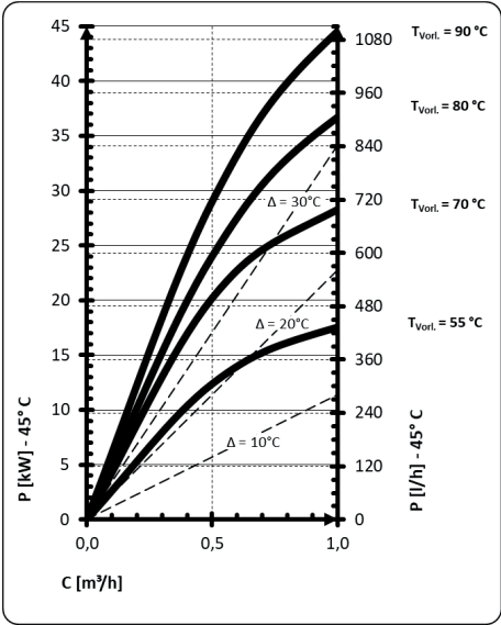
SPEICHER-LEISTUNGSDIAGRAMM
