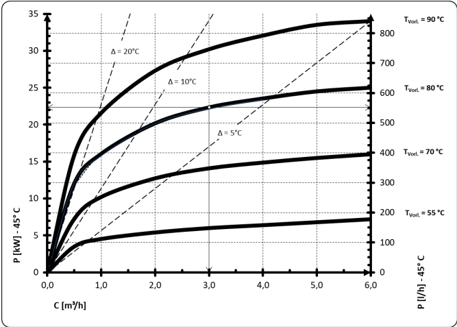
SPEICHER-LEISTUNGSDIAGRAMM
