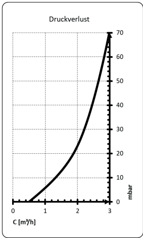
DRUCKVERLUST HEIZUNGSSEITE
