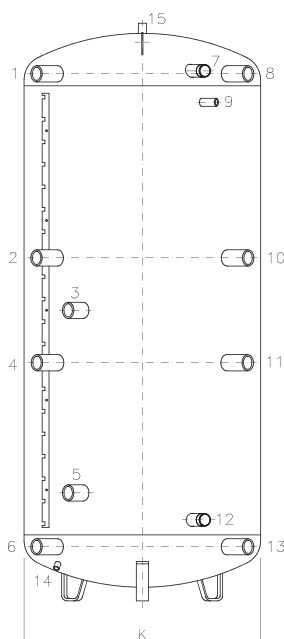
Vorderansicht
