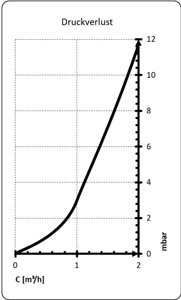
DRUCKVERLUST HEIZUNGSSEITE
