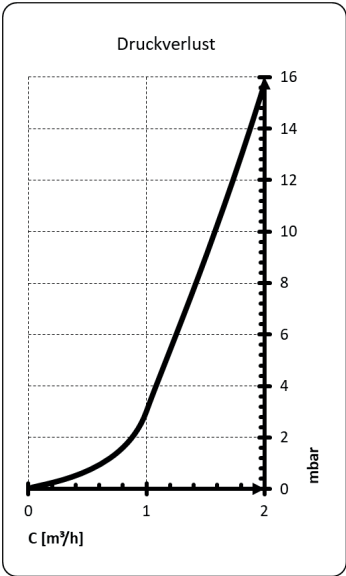
DRUCKVERLUST HEIZUNGSSEITE
