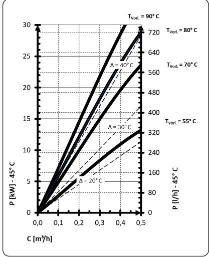
SPEICHER-LEISTUNGSDIAGRAMM
