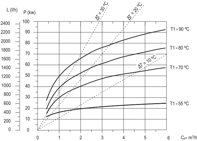
SPEICHER-LEISTUNGSDIAGRAMM
