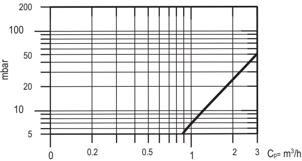
DRUCKVERLUST HEIZUNGSSEITE
