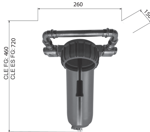
Abb. 44: Abmessungen AguaClean Home B L (MAXI) inklusive Moduluntertasse CLE U/Erweiterungs-Set CLE ES B (Zubehöre, nicht im Lieferumfang enthalten)
