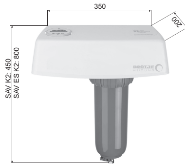
Abb. 40: Abmessungen AguaSave Home B inklusive Moduluntertasse SAV U/Erweiterungs-Set SAV ES K B (Zubehöre, nicht im Lieferumfang enthalten)
