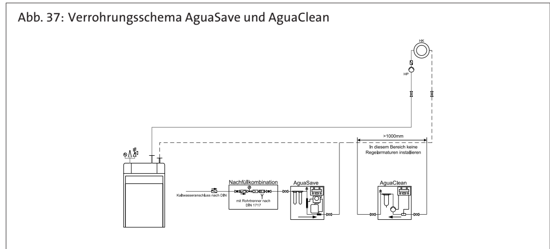
Abb. 38: Verrohrungsschema AguaSave Kompakt und AguaClean
