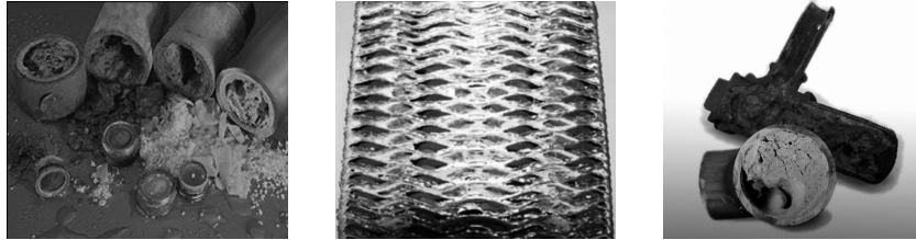
Abb. 3: Schäden im Heizungssystem
