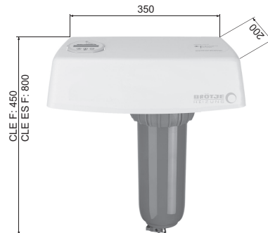
Abb. 45: Abmessungen AguaClean Home B inklusive Moduluntertasse CLE U/Erweiterungs-Set CLE ES B (Zubehöre, nicht im Lieferum- fang enthalten)
