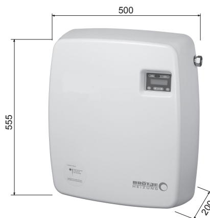
Abb. 41: Abmessungen AguaSave Kompakt (UMTS)
