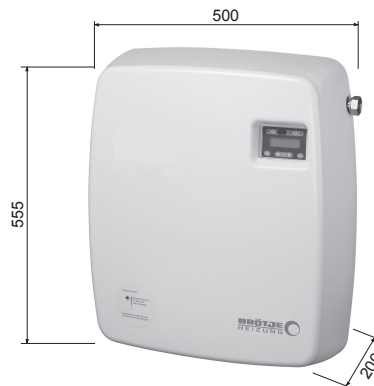
Abb. 46: Abmessungen AguaClean Kompakt
