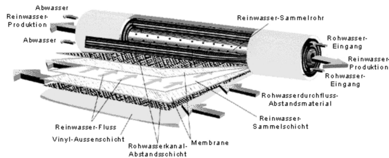
Abb. 8: Umkehrosmose
