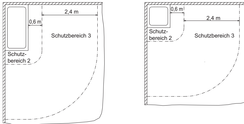
Abb 3: Abstände WBS in Bad- bzw. Duschräumen
