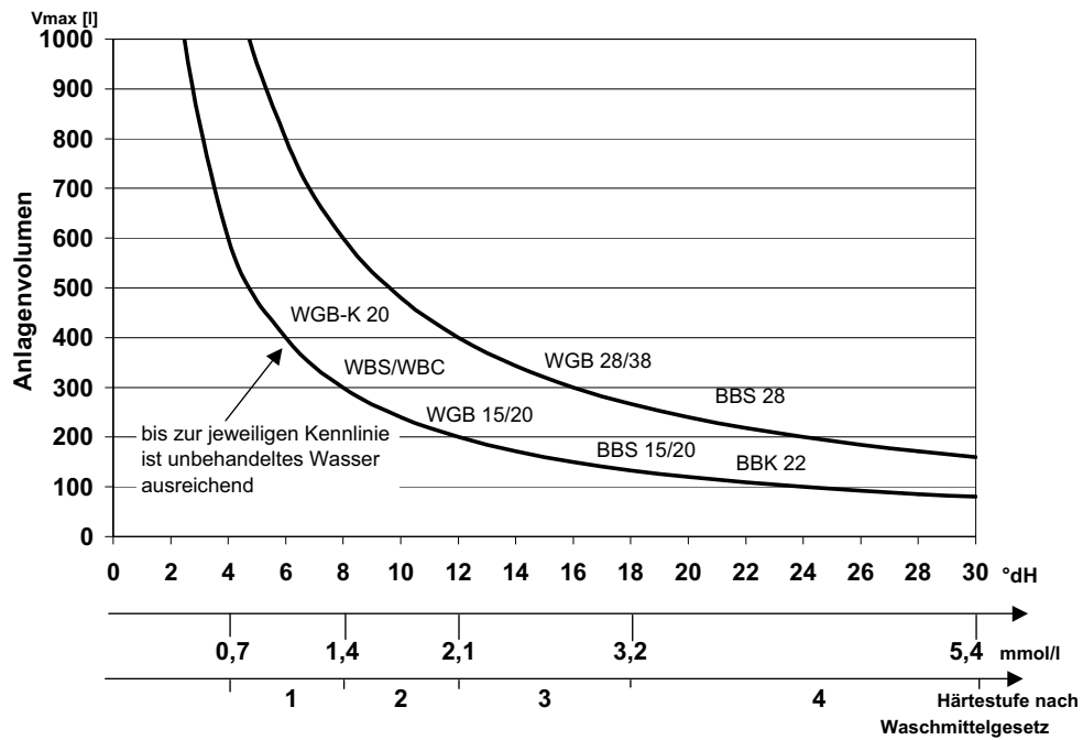
Abb 2: Diagramm Wasserhärte
