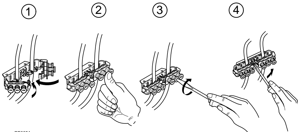
Abb 9: Zugentlastung
