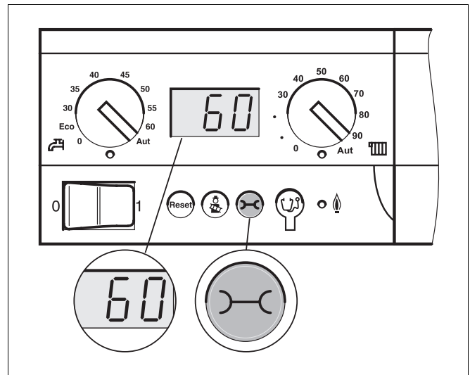
Bild 9 Taste „Statusanzeige“
