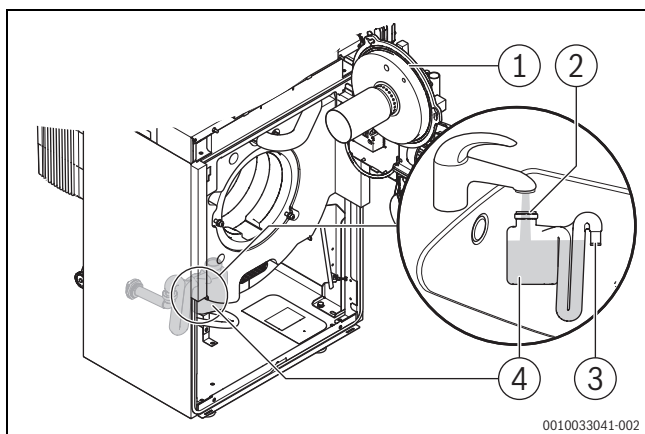
Bild 78 Siphon reinigen
