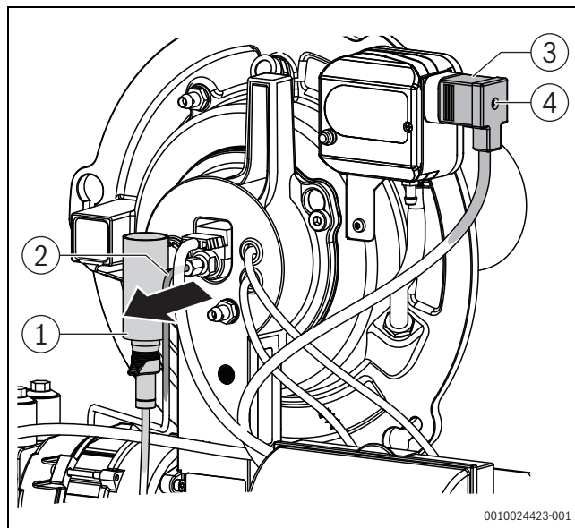
Bild 67 Ölleitung herausziehen
