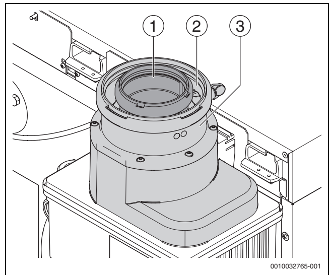
Bild 16 Abgasanschluss montieren
