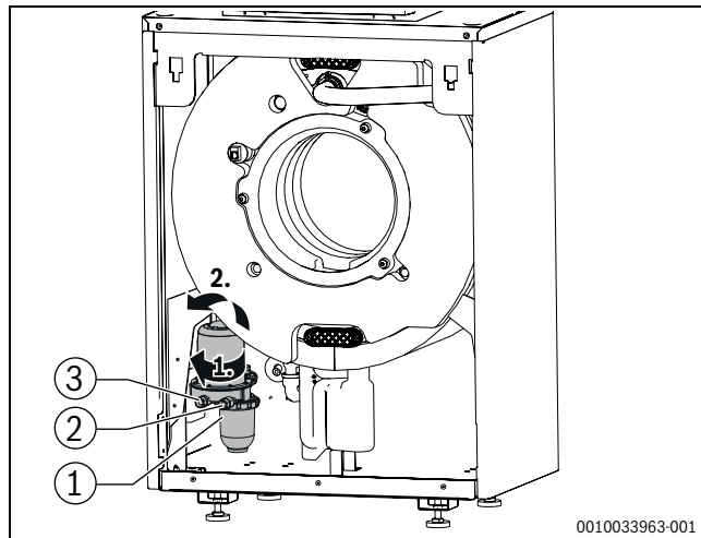
Bild 72 Ölfilter demontieren
