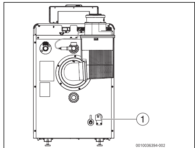
Bild 29 Haltewinkel montieren
