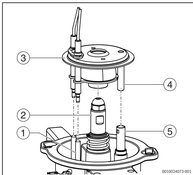
Bild 65 Mischsystem montieren
