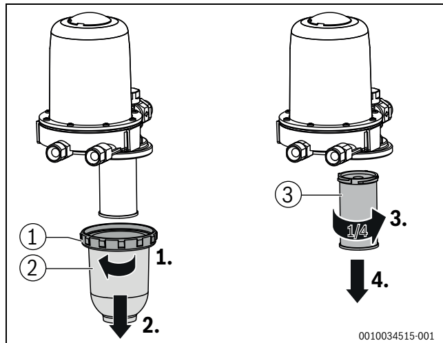
Bild 73 Filtertasse entfernen
