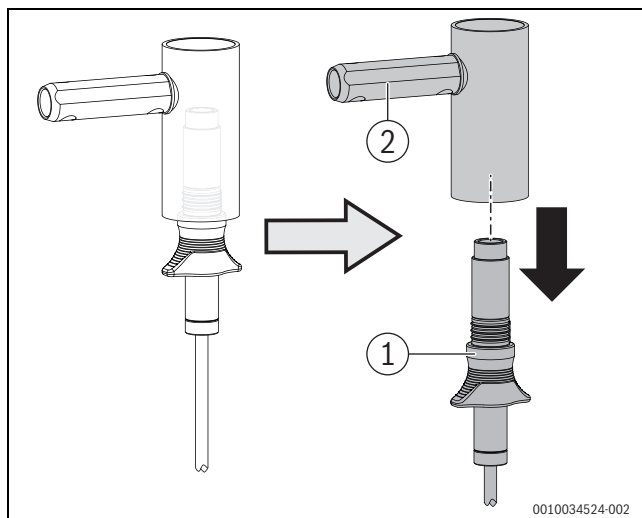
Bild 81 Flammenfühler demontieren
