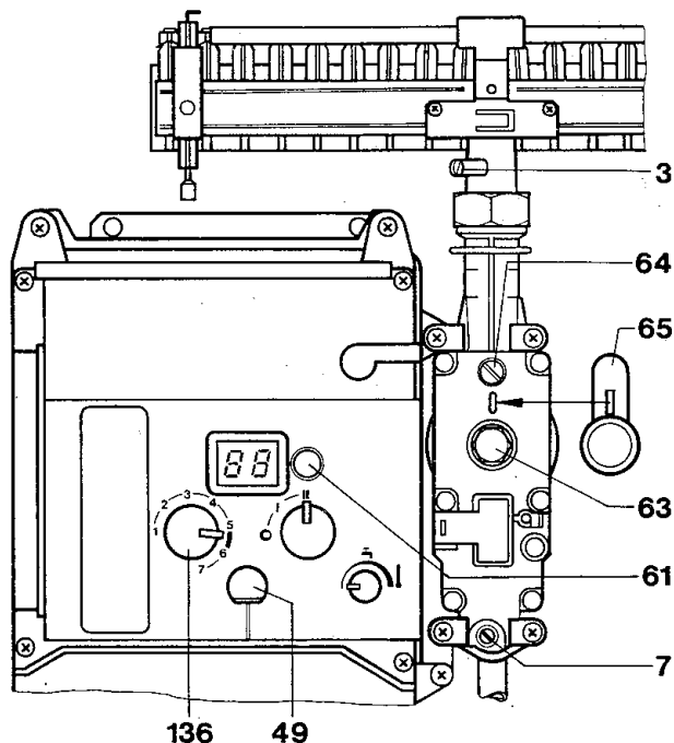
Bild 30 Gasarmatur CE 426, Erd- und Flüssiggas
