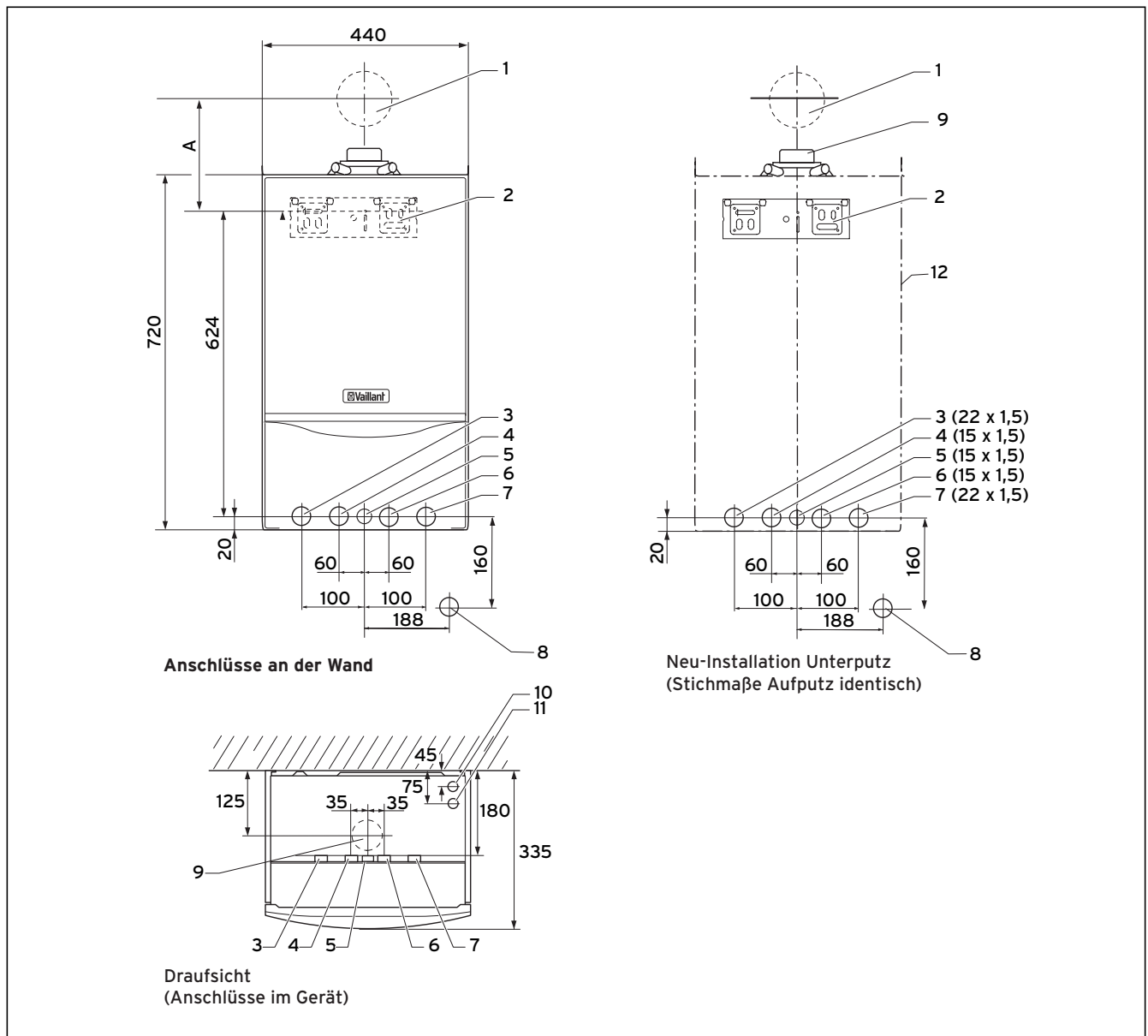
Abb. 4.3 Anschlussmaße in mm (VCW-Geräte)
