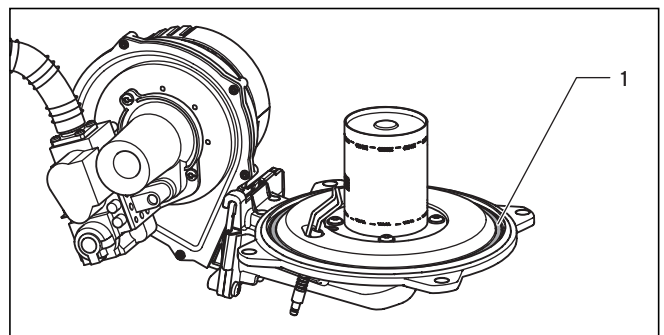
Abb. 8.5 Brennertürdichtung ersetzen
