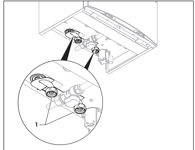
Abb. 5.3 Speicheranschluss montieren
