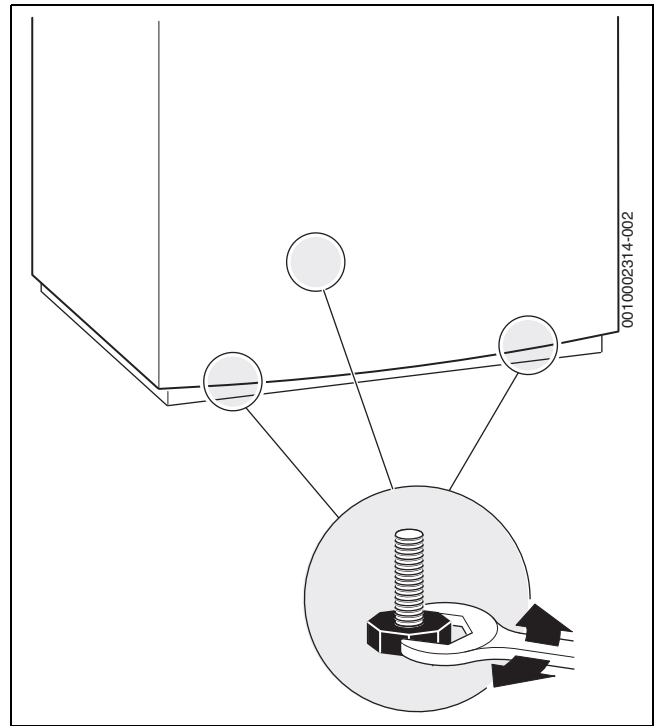
Bild 50 Speicher ausrichten
