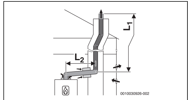
Bild 33 Flexible Abgasführung im Schacht nach B 23p /B 53p mit raumluftabhängiger Luftzufuhr am Gerät und konzentrischem Verbindungsstück zwischen Aufstellraum und Schacht
