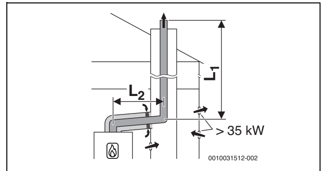
Bild 34 Starre Abgasführung im Schacht nach B 33 mit raumluftabhängiger Luftzufuhr über die konzentrische Luft-Abgas-Führung im Aufstellraum
