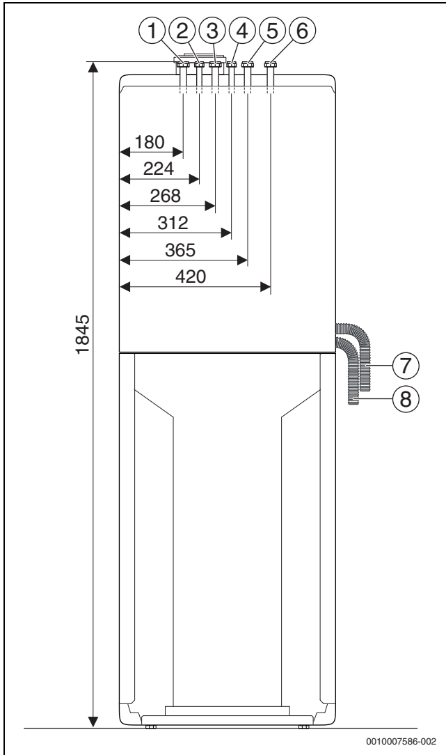
Bild 7 Anschlussmaße des Zubehörs AS-V1/Vertikales Anschluss-Set (Maße in mm)
