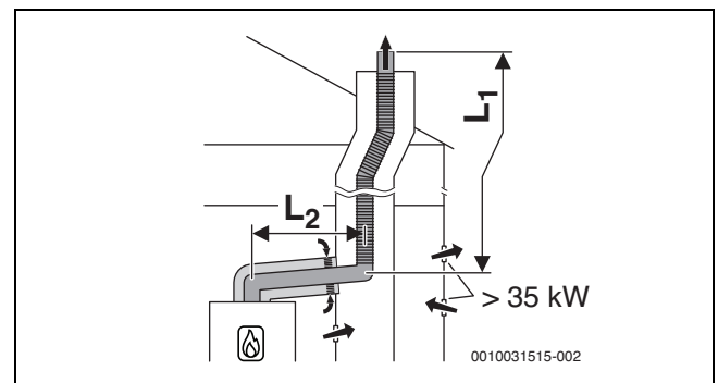
Bild 35 Flexible Abgasführung im Schacht nach B 33 mit raumluftabhängiger Luftzufuhr über die konzentrische Luft-Abgas-Führung im Aufstellraum
