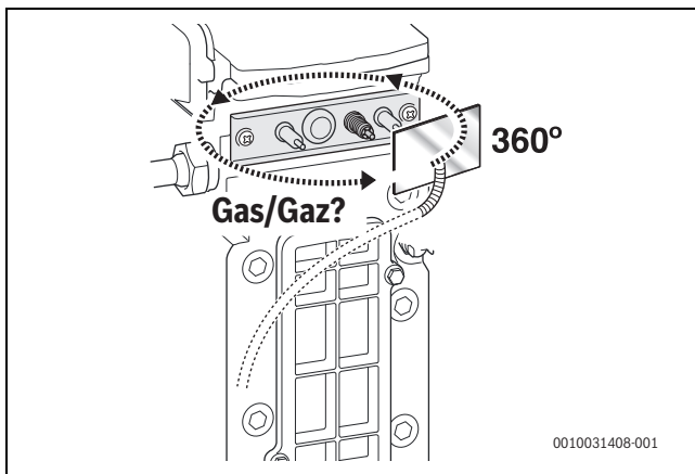
Bild 202 Dichtheit kontrollieren
