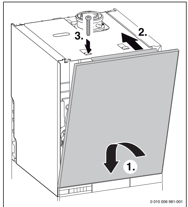
Bild 189 Vordere Verkleidung einhängen und mit Schraube aus Lieferumfang sichern
