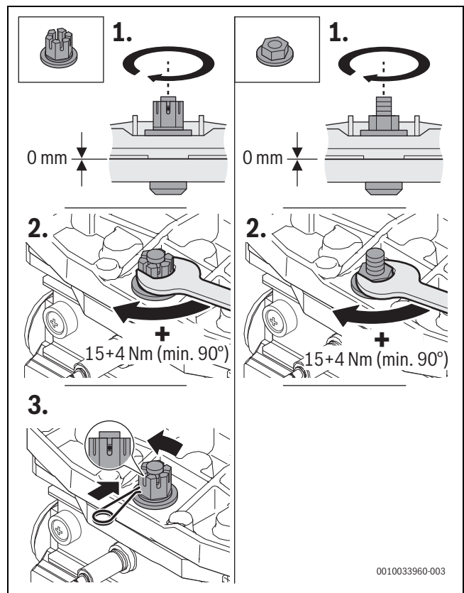
Bild 205 Mutter am Brennerdeckel festziehen
