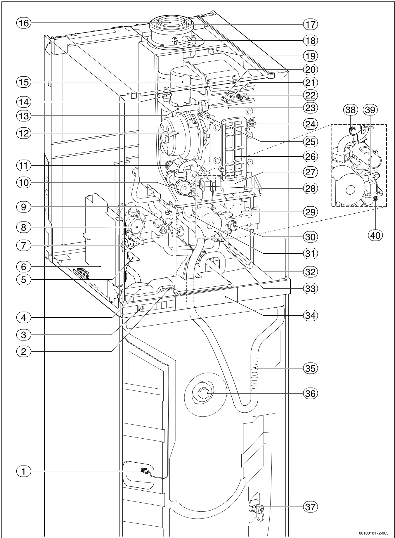
Bild 16 GB192-..iT150..-Geräte
