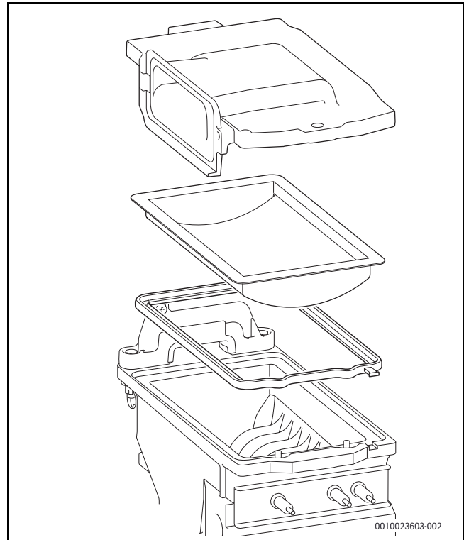
Bild 204 Brenner
