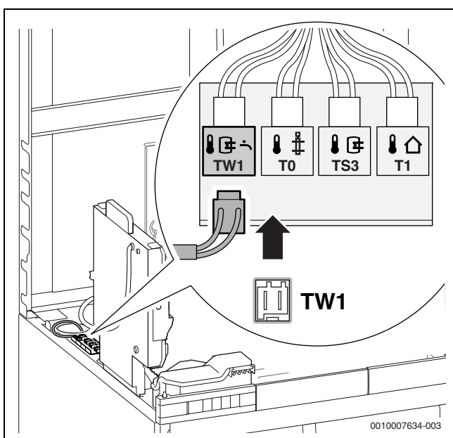
Bild 62 Speichertemperaturfühler anschließen
