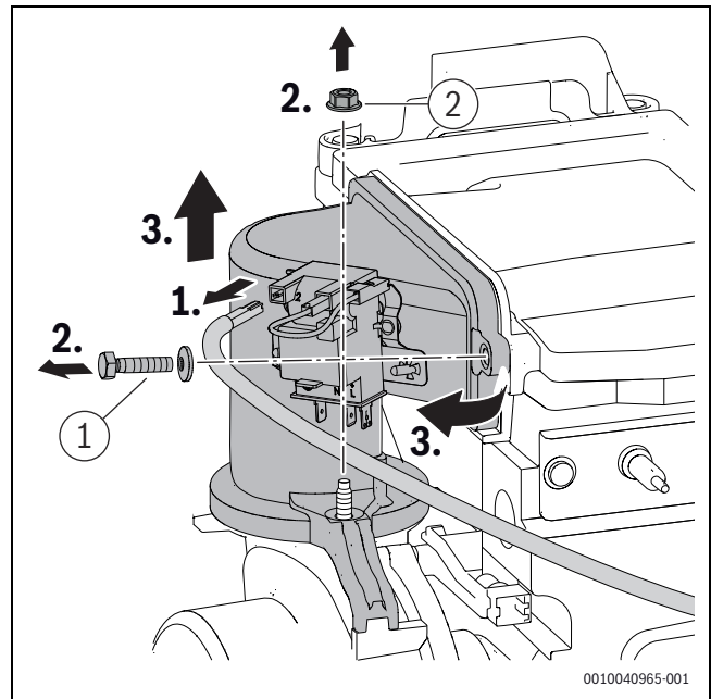
Bild 212 Mischeinrichtung ausbauen
