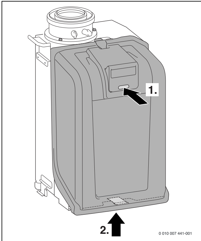
Bild 195 Brennerhaube abnehmen
