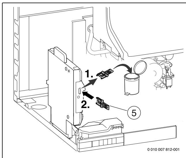
Bild 141 KIM tauschen
