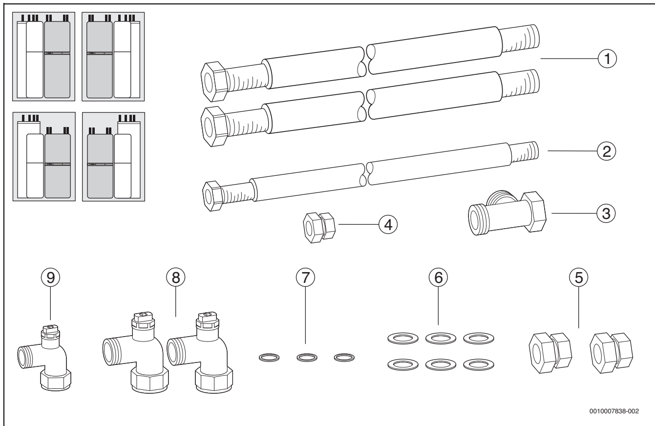
Bild 170 Lieferumfang
