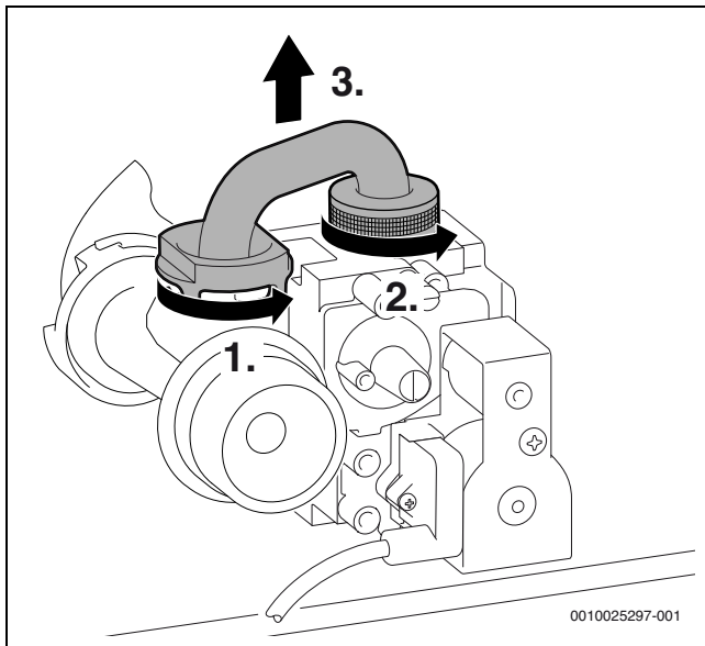
Bild 215 Gasrohr ausbauen
