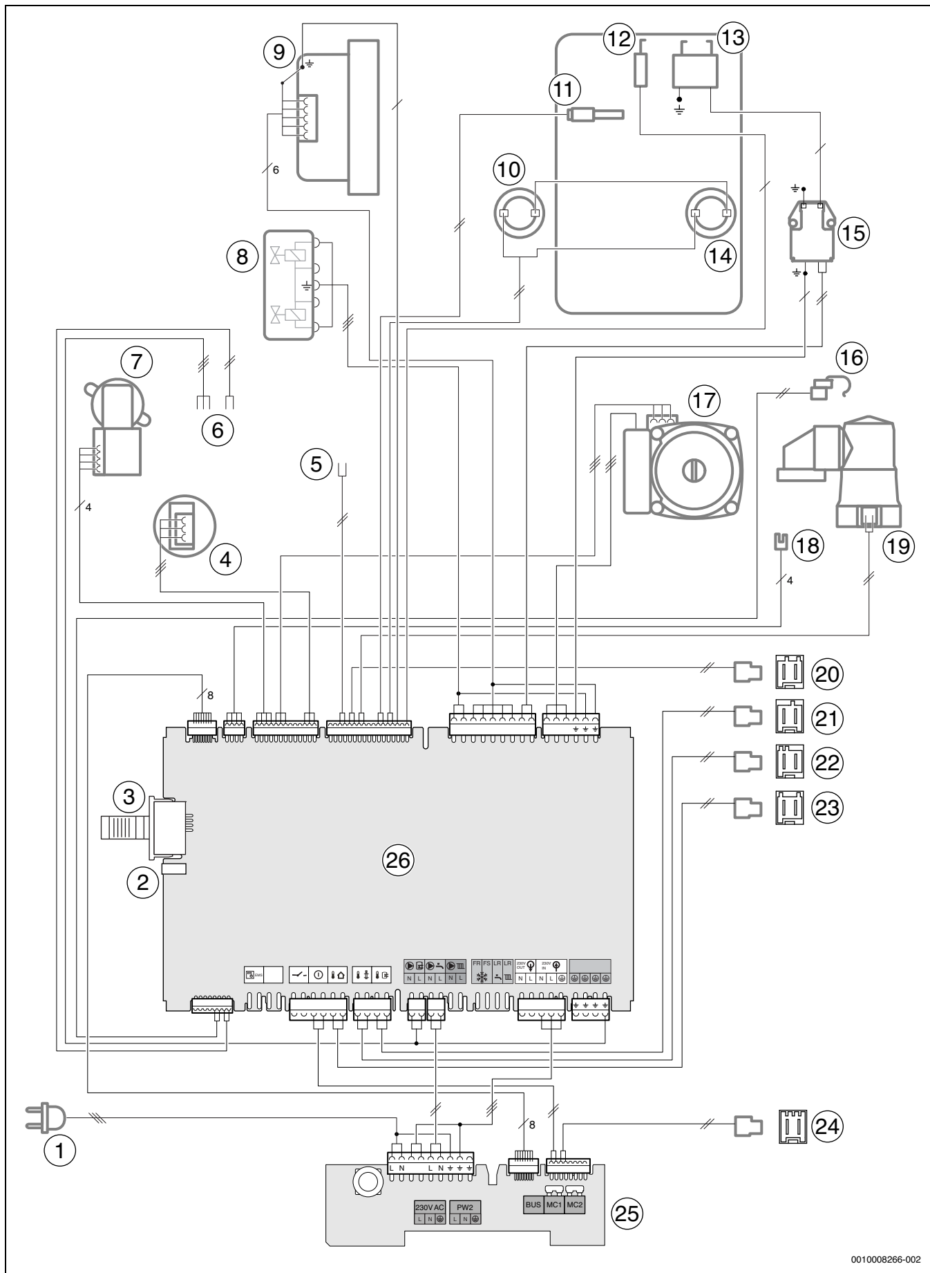
Bild 221 Elektrische Verdrahtung
