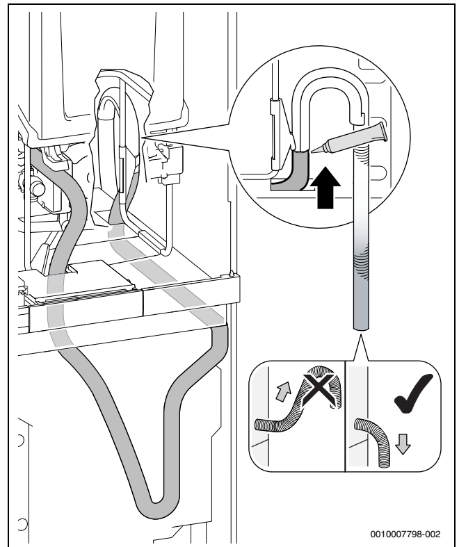
Bild 55 Siphonschlauch am Endstück einstecken
