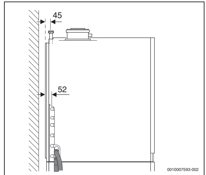
Bild 10 Anschlussmaße des Zubehörs Heizkreiserweiterung 1 (Maße in mm)
