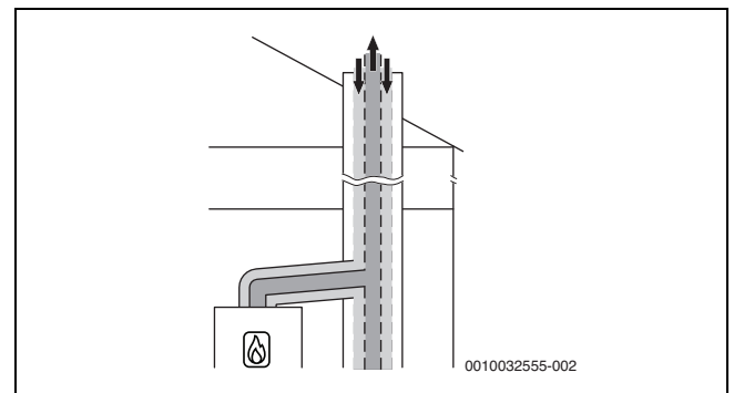
Bild 26 Konzentrische Luft-Abgas-Führung nach C 43x im Aufstellraum
