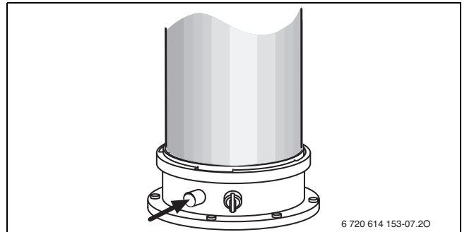
Bild 197 Abgasmessstutzen
