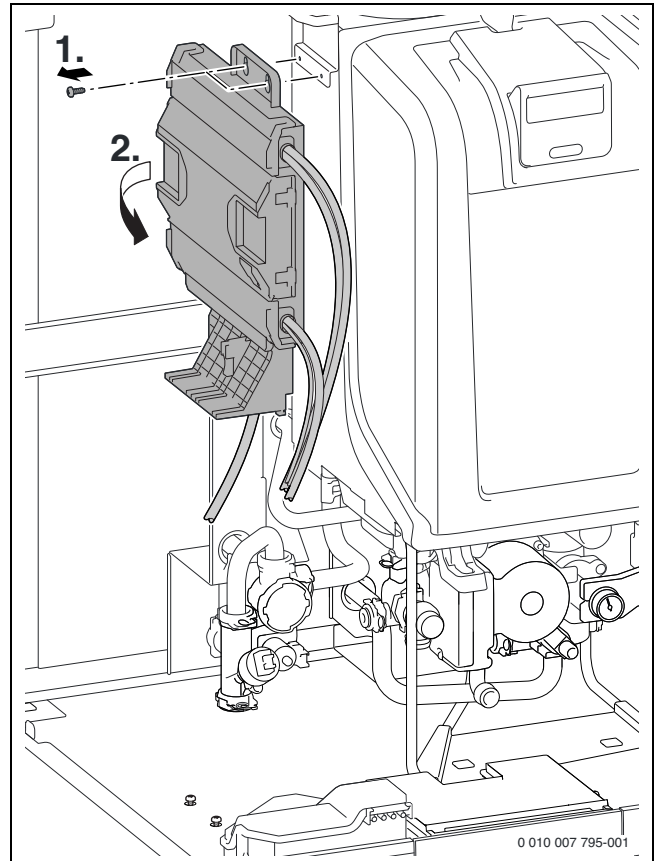
Bild 59 Steuergerät abnehmen
