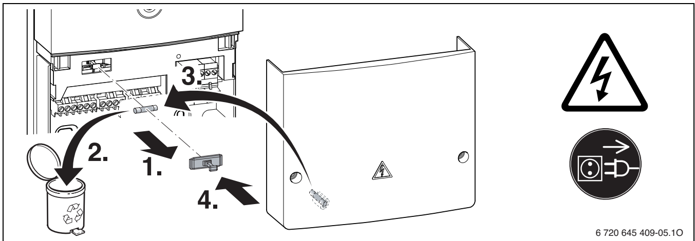
Bild 220 Sicherung vom Modul tauschen
