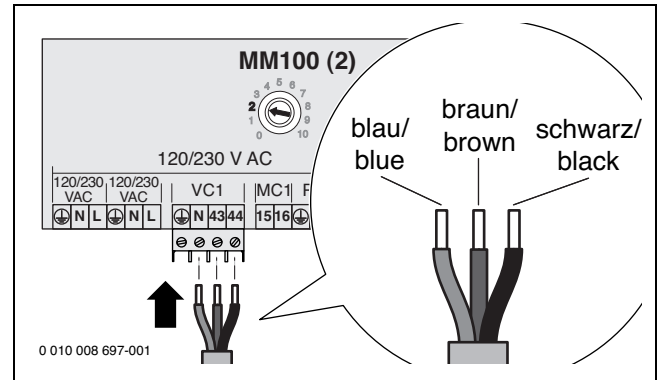
Bild 136 Anschluss Kabel Mischemotor am Modul MM100 [2]
