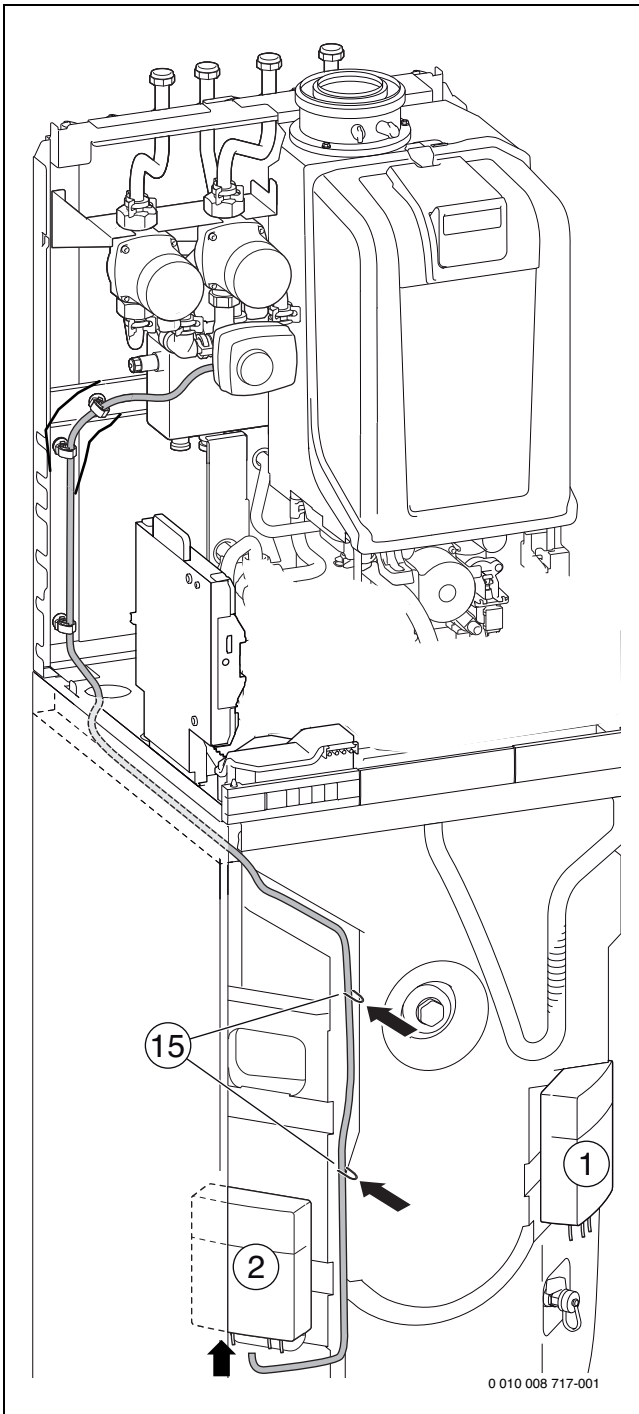
Bild 134 Anschluss Mischemotor
