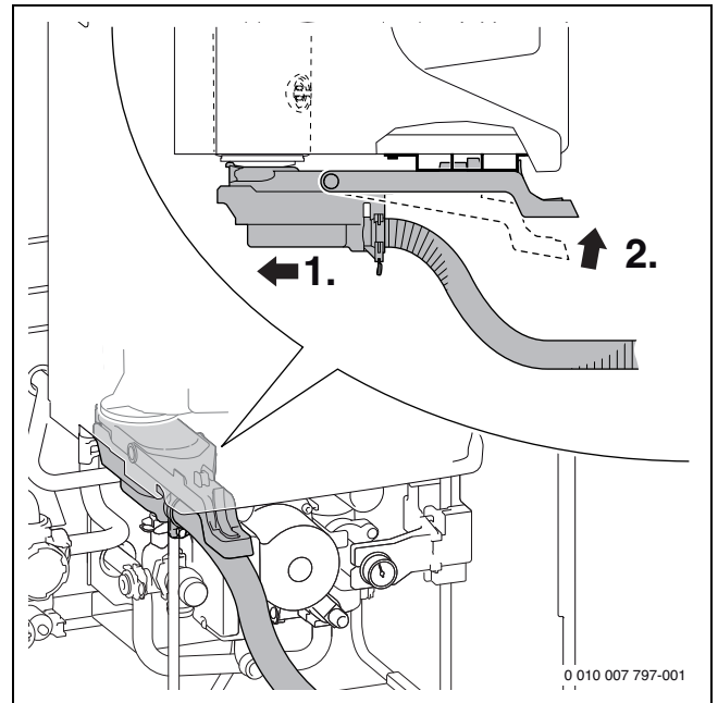
Bild 54 Schmutzfänger montieren
