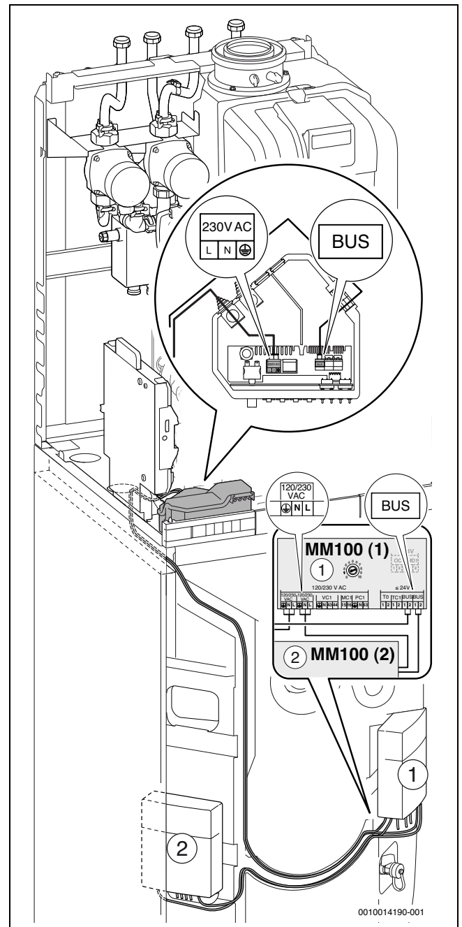
Bild 137 Anschluss MM100 (1) und MM100 (2)
