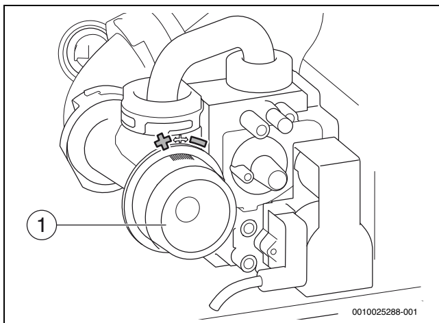
Bild 196 Gas-Luft-Verhältnis einstellen
