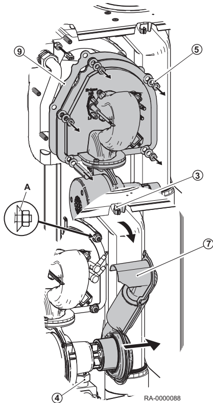
Abb.45 Gasbrenner ausbauen
