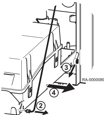
Abb.42 Kesselschaltfeld aushaken
