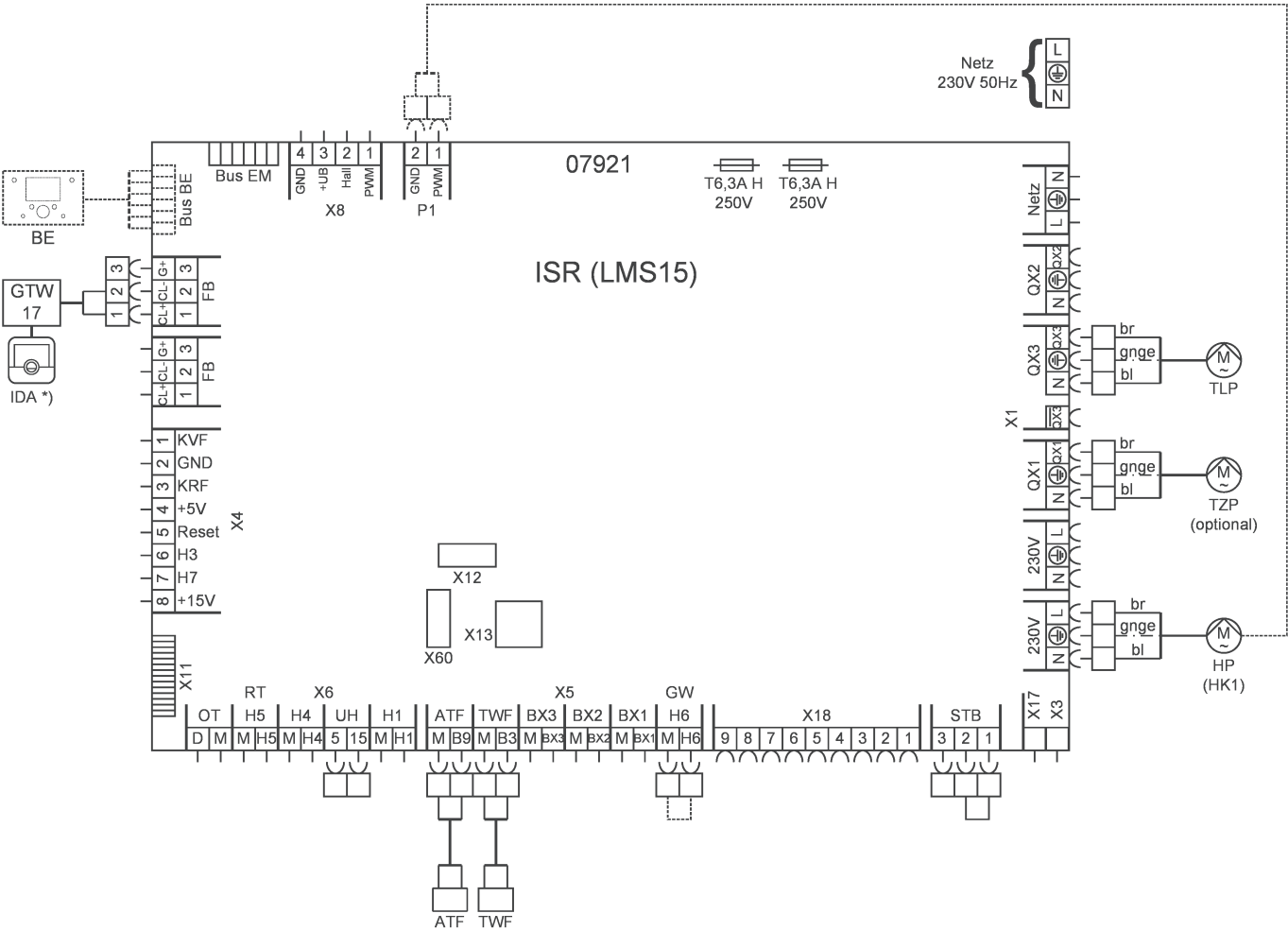
Abb.13 Anschlussplan
