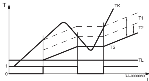
Abb.37 Laderegelung /schematisch)
