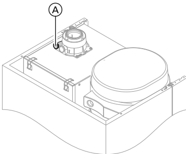
(A) Verbrennungsluftöffnung
