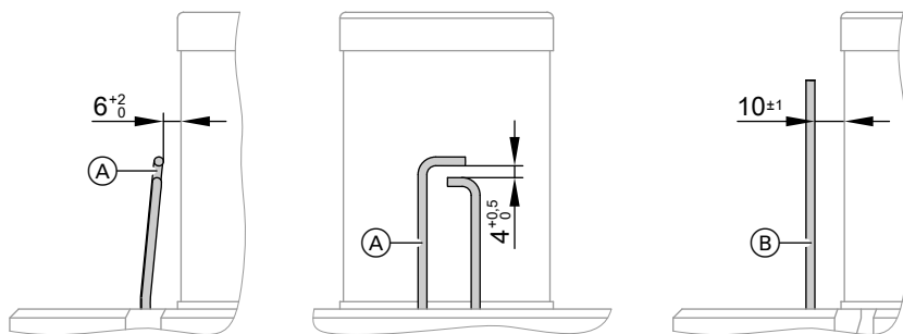
(A) Zündelektroden
