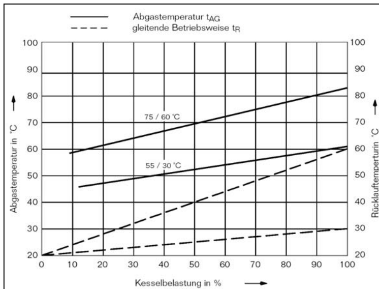
Abgastemperaturen und Rücklauftemperaturen in Abhängigkeit von der Kesselbelastung
