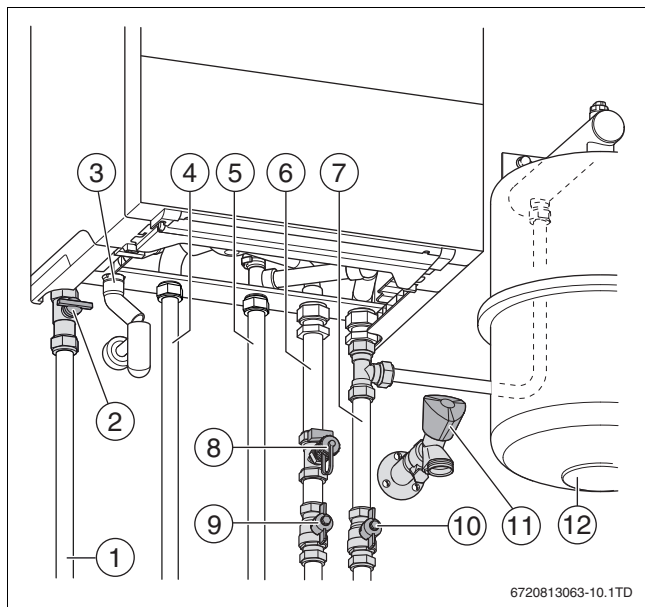
Bild 1 Anschlusszubehör (Beispiel)
