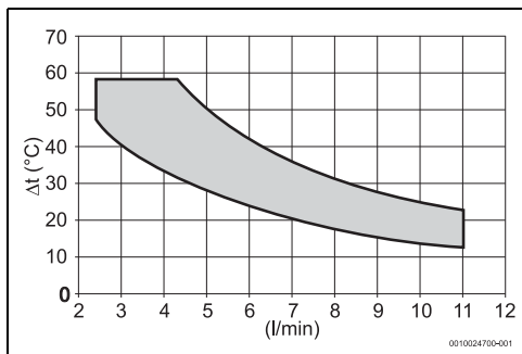
Bild 24 10-Liter-Modell
