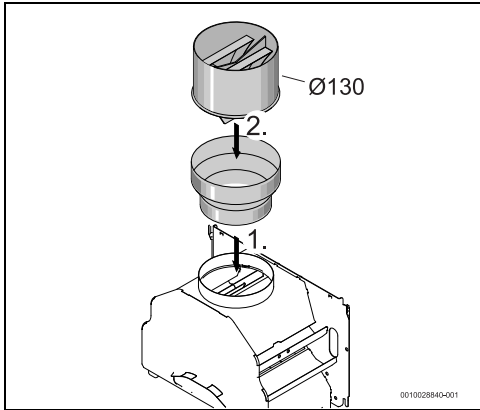
Bild 10 Ø 130 mm montieren
