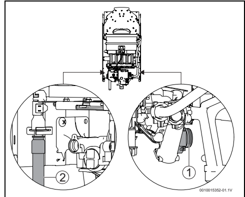
Bild 11 Wasseranschluss
