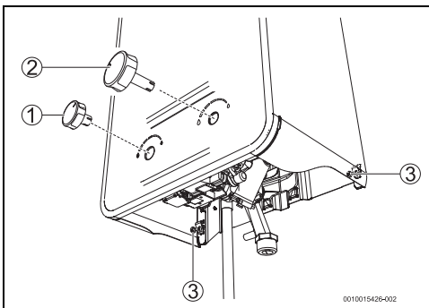
Bild 14 Verkleidung entfernen
