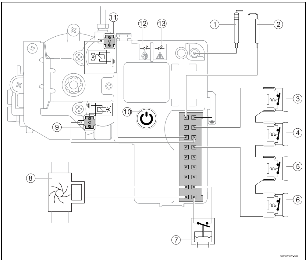
Bild 23 Schaltplan
