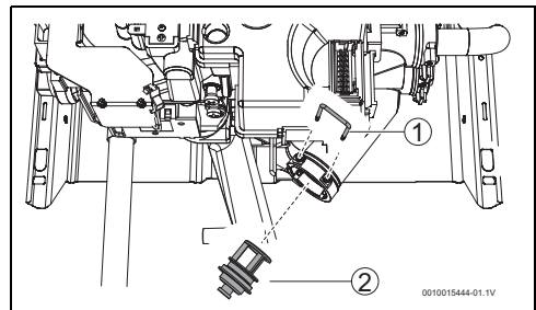
Bild 8 Entleeren
