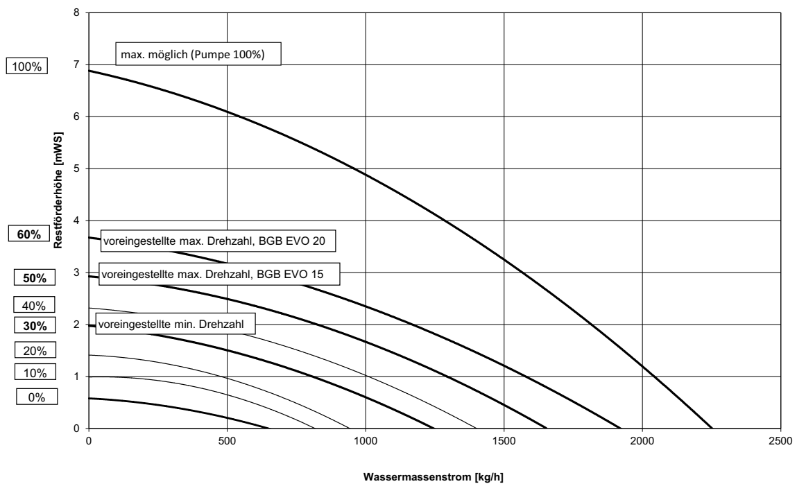
Abb. 8: Restförderhöhe Pumpenheizkreis BGB EVO 15/20 i
