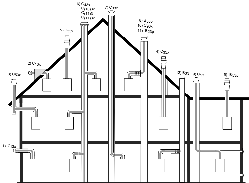
Abb. 12: KAS 60 und KAS 80
