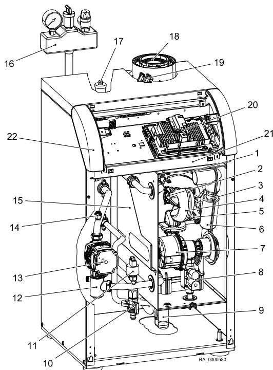
Abb. 1: BGB EVO 15–38 i (dargestellt ohne Vorderwand und Abdeckung der Regelung)
