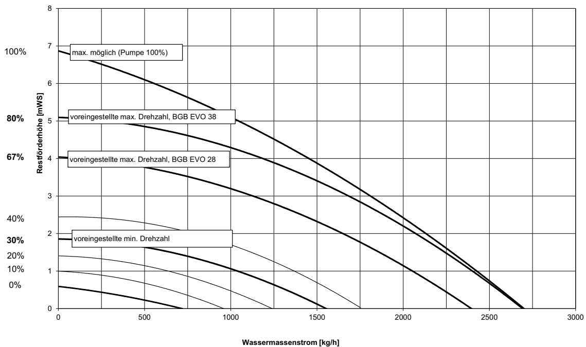
Abb. 9: Restförderhöhe Pumpenheizkreis BGB EVO 28/38 i
