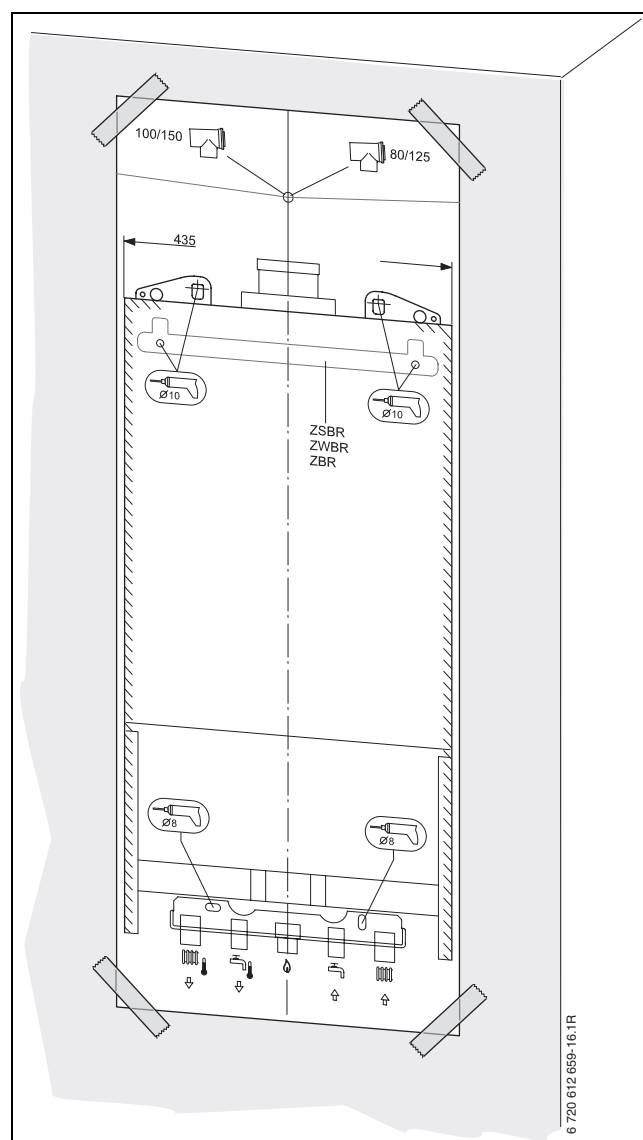
Bild 10 Montageschablone
