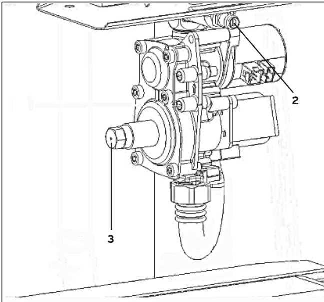
Abb. 6.3 Nennbelastung einstellen
