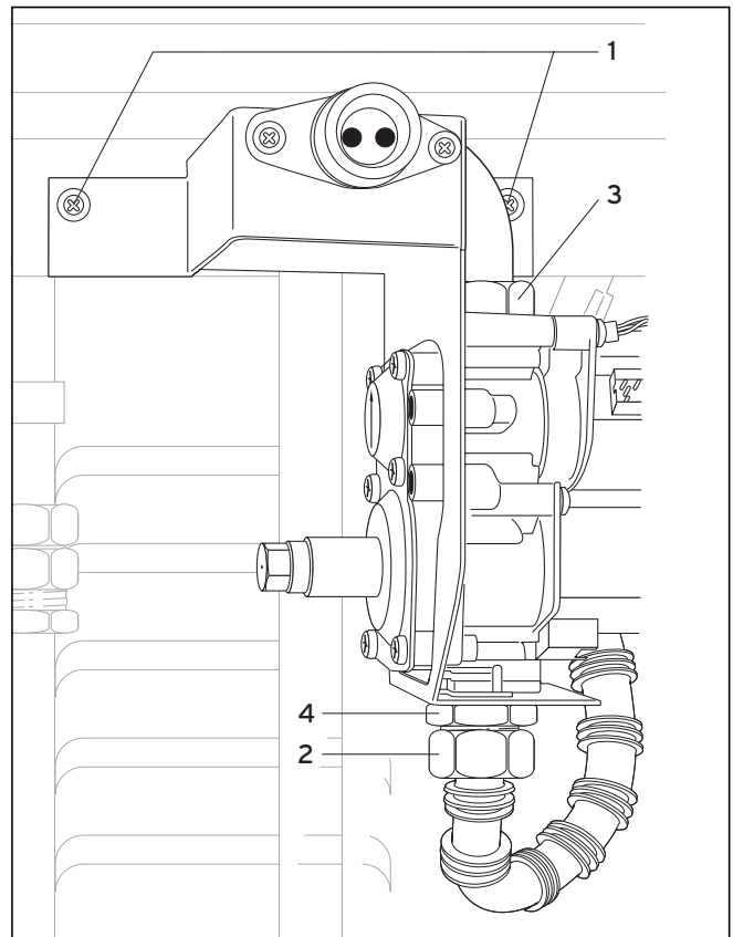
Abb. 9.3 Austauschen der Gasarmatur
