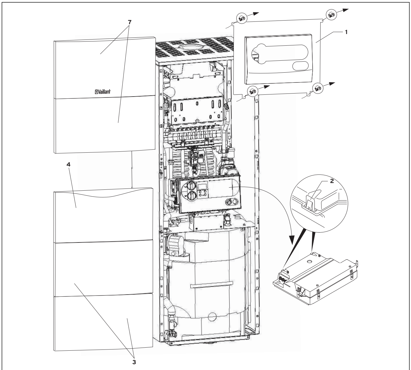
Abb. 5.3 Geräteverkleidungen abnehmen
