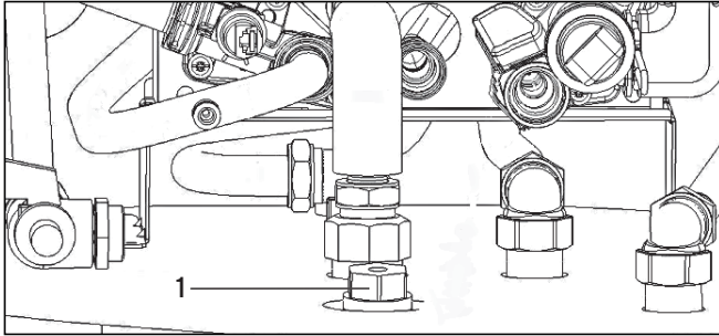
Abb. 8.8 Magnesium-Schutzanode warten
