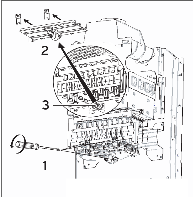
Abb. 9.2 Brennerdüsen ausbauen
