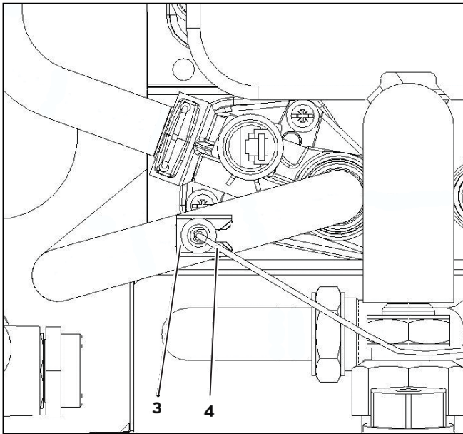
Abb. 9.6 Anschluss-Stutzen für Kapillarrohr
