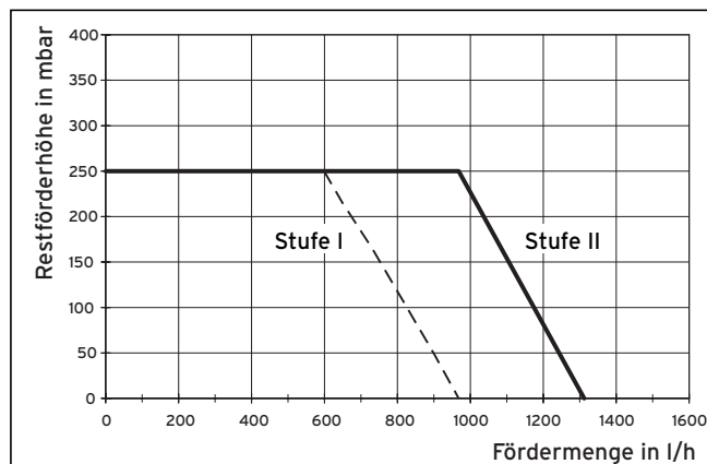
Abb. 7.2 Pumpenkennlinie VSC
