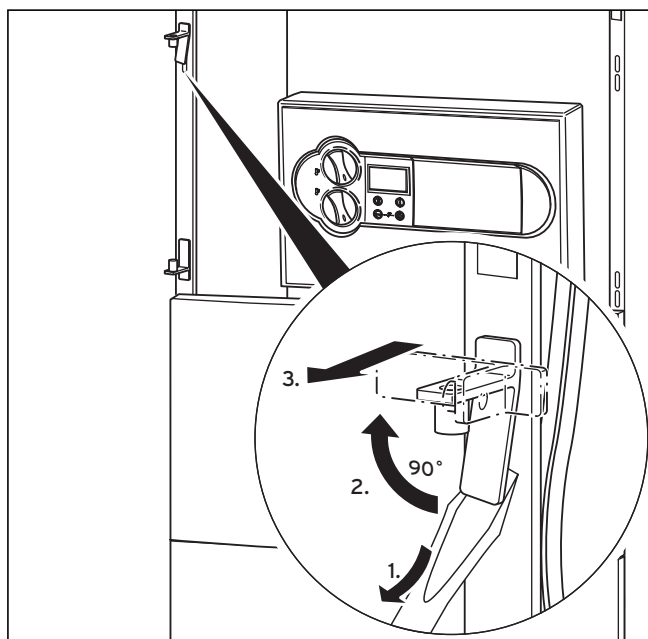
Abb. 4.10 Türanschlag wechseln
