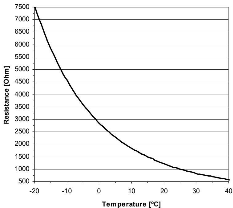
NTC 1k \Omega Temperatursensor (Aussenfühler)
