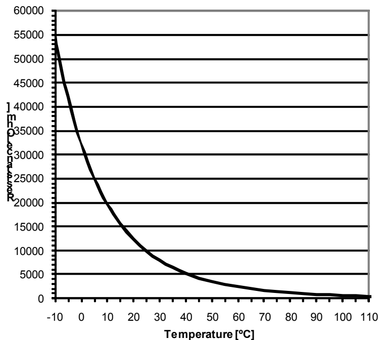
NTC 10k \Omega Temperatursensor (Vorlauf-, Rücklauf-, Abgas-, Brauchwasser- und Weichefühler)
