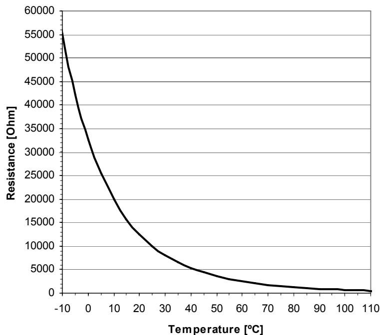
NTC 10k \Omega capteur de température (de temperature debit/retour eau, gaz brûlés, ECS et tuyau collecteur )
