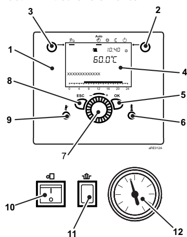
Abb.2 Bedienelemente
