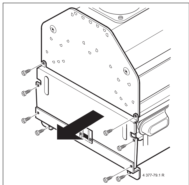
Bild 54 ZWR/ZSR 18/24...-7 KE..
