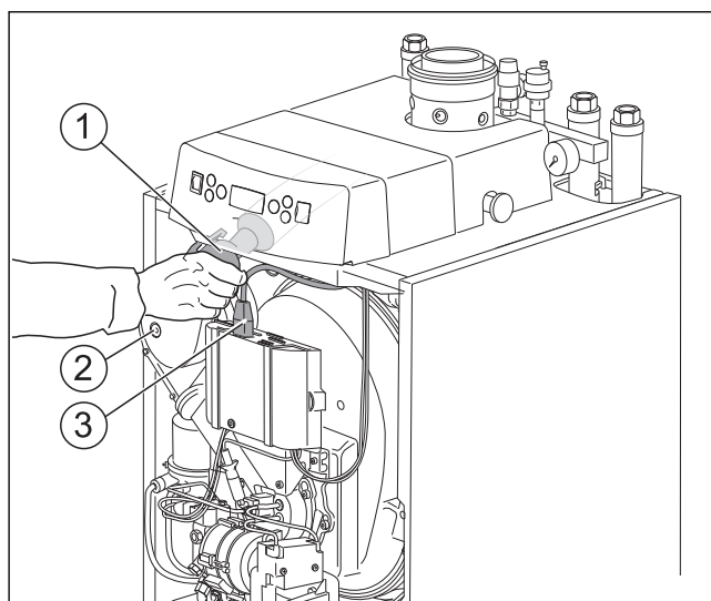
Bild 52 Venturi abnehmen
