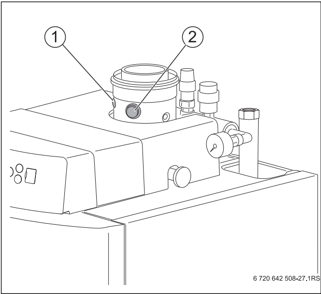
Bild 45 Messwerte aufnehmen
