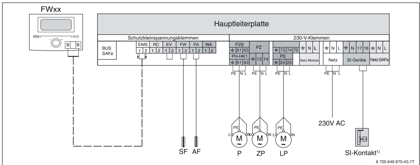
Bild 15 Anschluss ungemischter Heizkreis mit Warmwasserbereitung über Kesselregelung
