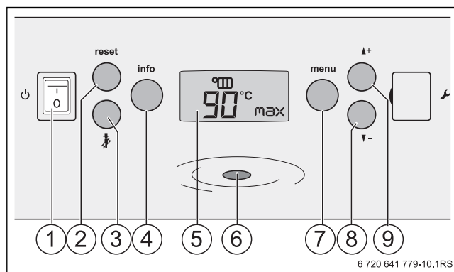
Bild 38 Bedienelemente
