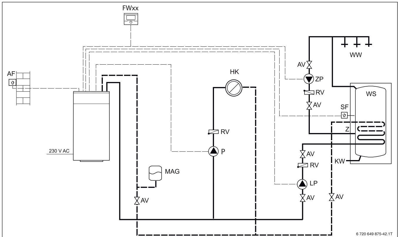
Bild 14 Vereinfachtes Anlagenbeispiel: Ein ungemischter Heizkreis mit Warmwasserbereitung über Kesselregelung
