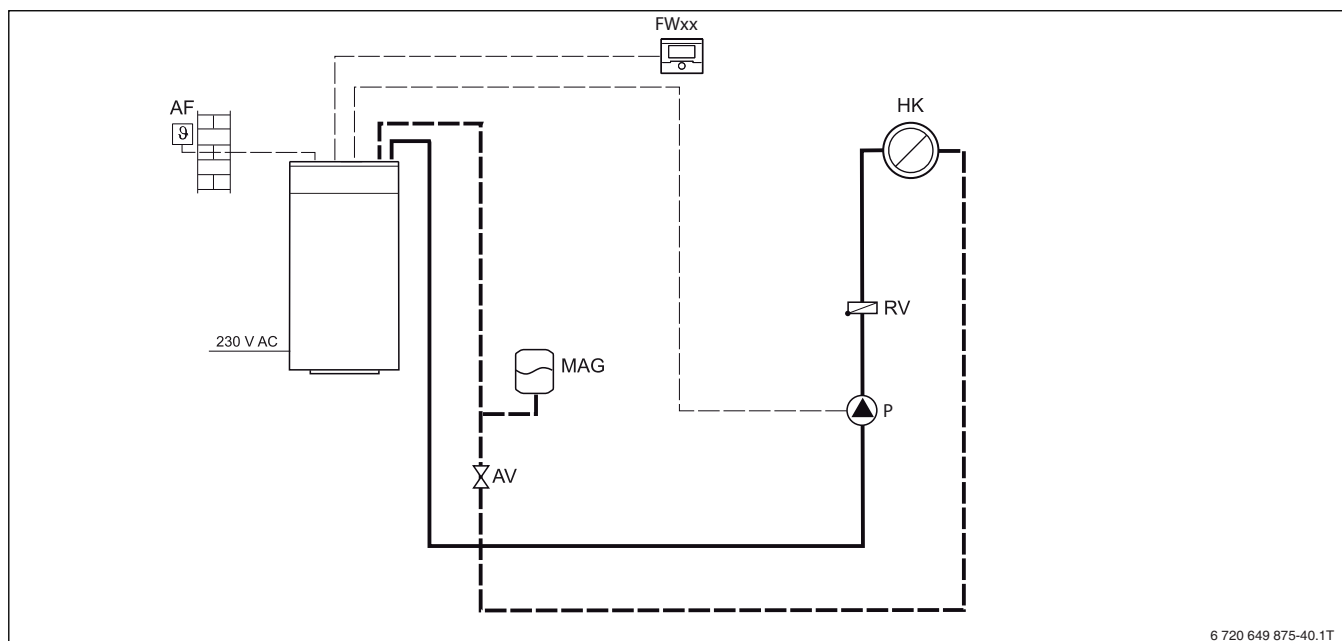
Bild 12 Vereinfachtes Anlagenbeispiel: Ein ungemischter Heizkreis
