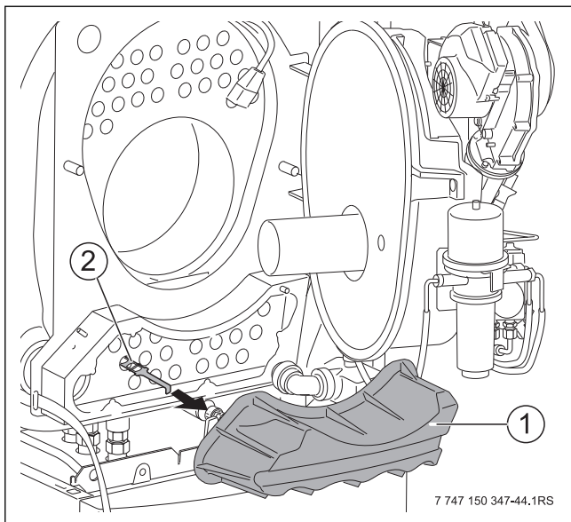
Bild 67 Turbulatoren herausziehen
