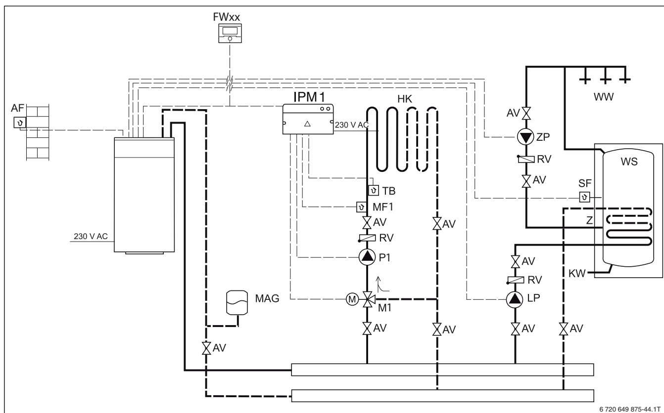
Bild 16 Vereinfachtes Anlagenbeispiel: Ein gemischter Heizkreis und Warmwasserbereitung über Kesselregelung
