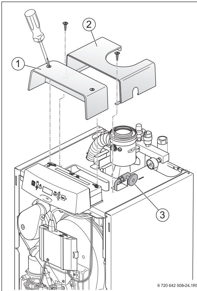
Bild 32 Ölleitung anschließen
