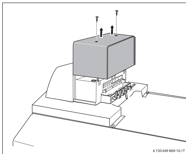
Bild 35 Abdeckhaube abnehmen
