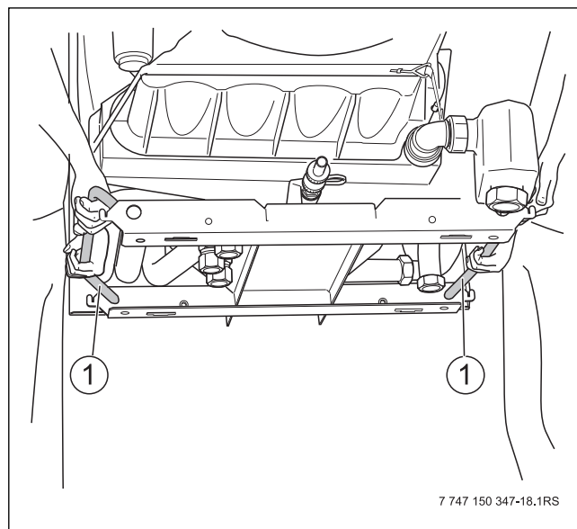
Bild 11 Heizkessel heben und tragen
