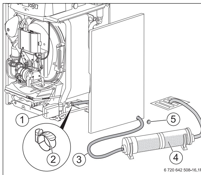
Bild 25 Kondensatablauf mit Neutralisation
