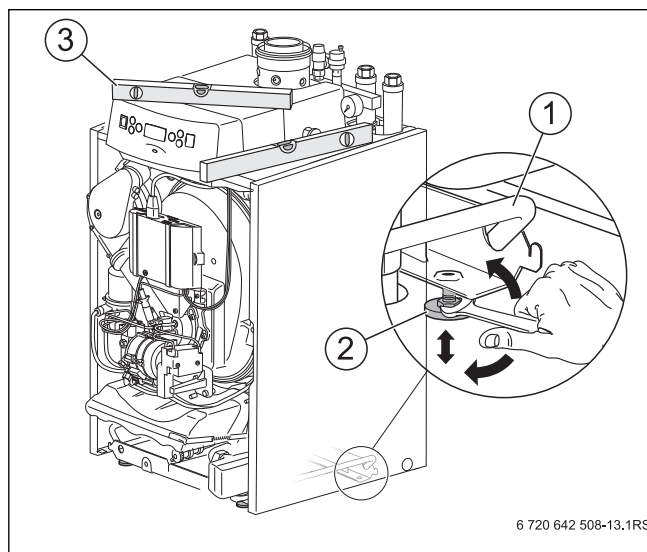
Bild 24 Heizkessel ausrichten
