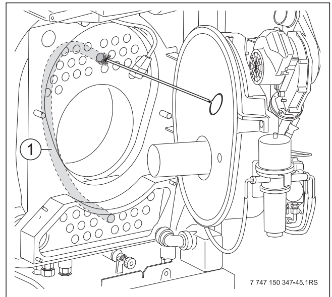
Bild 68 Heizgaszüge reinigen
