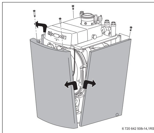
Bild 10 Seitenwände abnehmen
