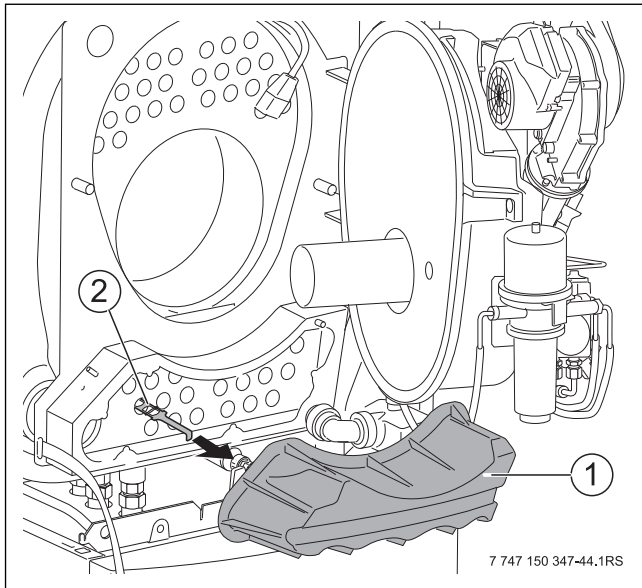
Bild 69 Turbulatoren herausziehen
