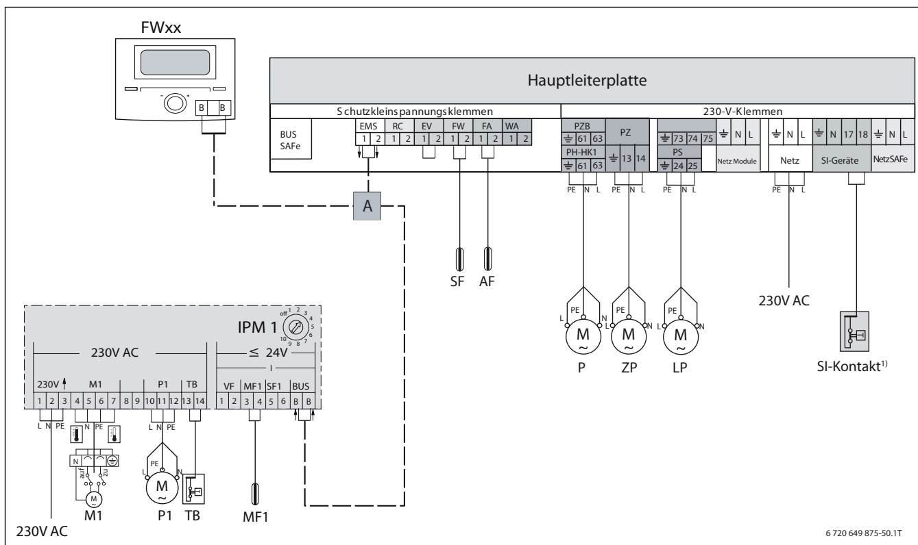
Bild 19 Anschlussplan gemischter Heizkreis und ungemischter Heizkreis mit Warmwasserbereitung über Kesselregelung
