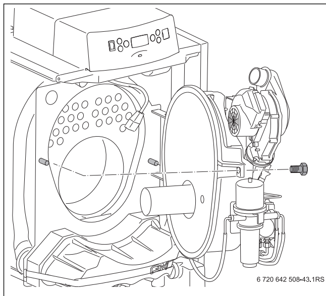
Bild 65 Brenntür öffnen
