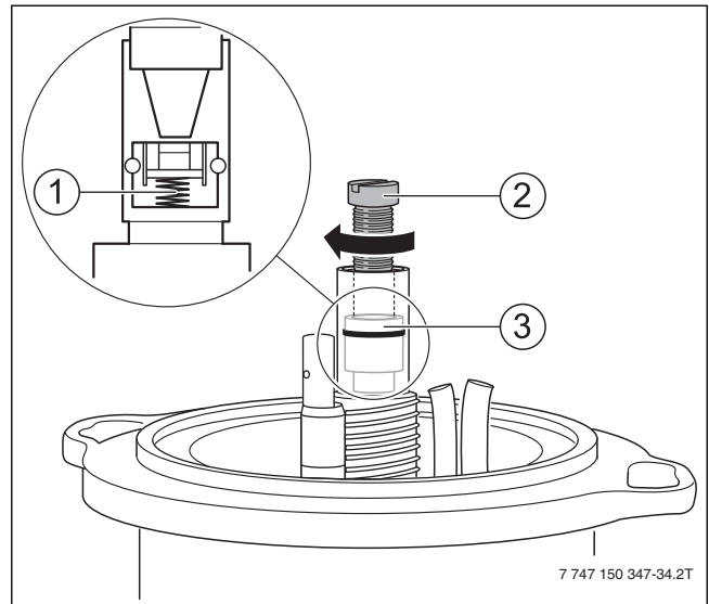
Bild 59 Abschlussventil austauschen
