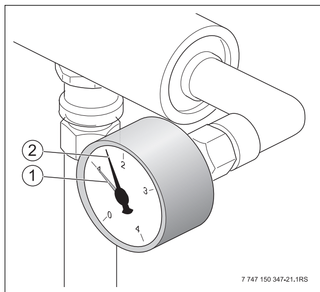
Bild 27 Manometer
