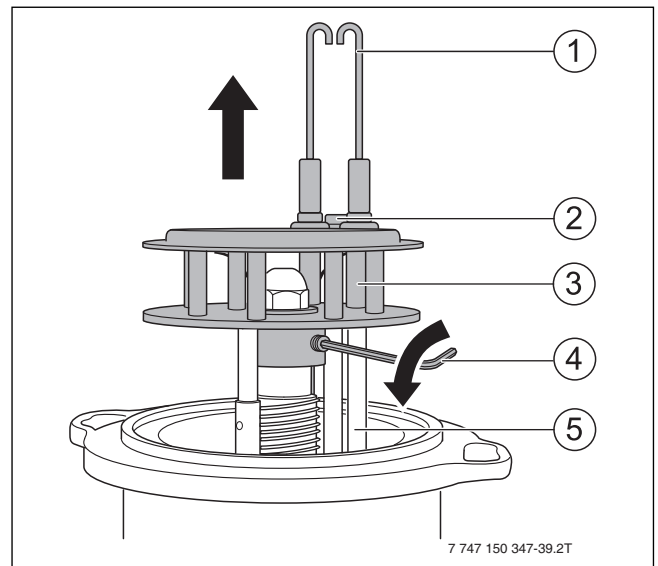
Bild 76 Mischsystem ausbauen
