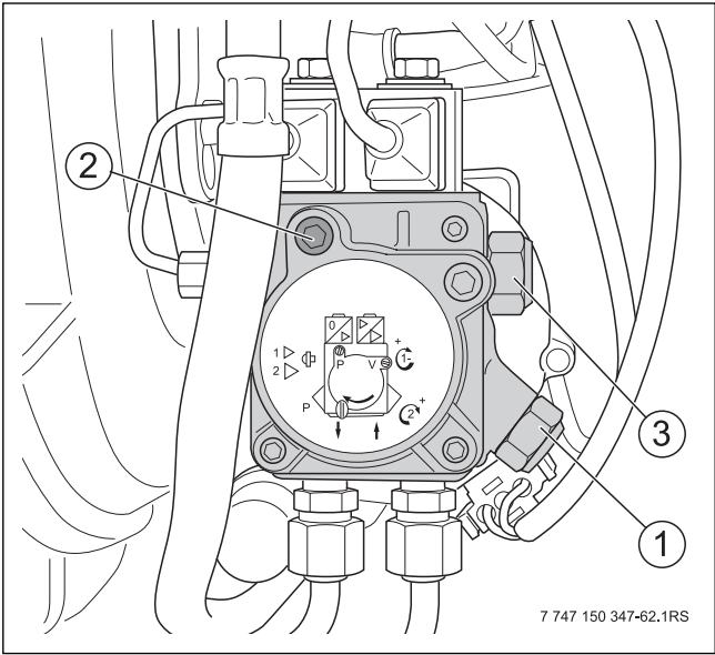
Bild 46 Druck einstellen
