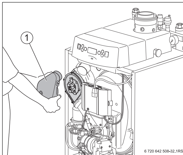
Bild 53 Verbrennungsluftanschluss abnehmen
