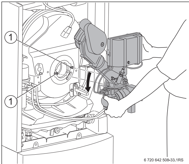
Bild 74 Brenner herausnehmen
