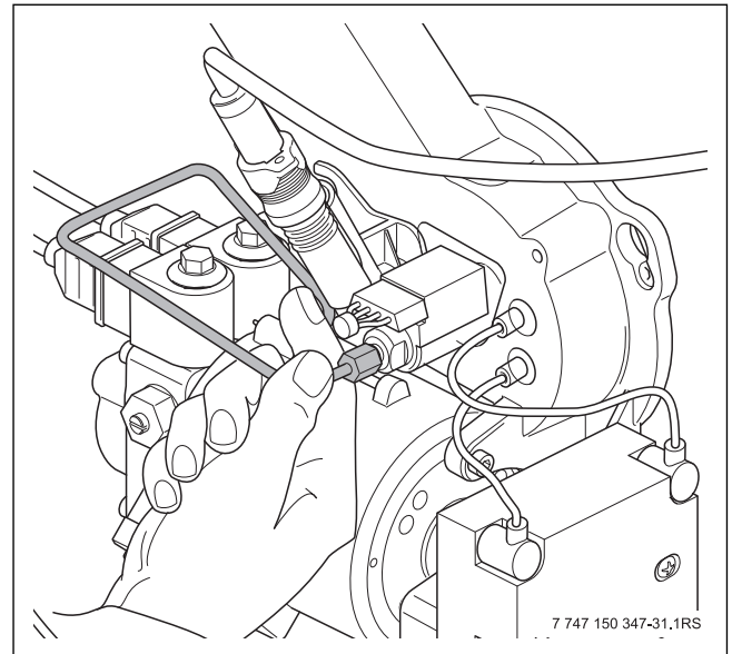
Bild 63 Ölleitung herausziehen
