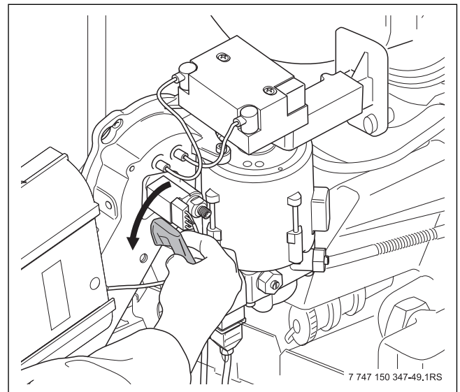
Bild 77 Winkelhalter demontieren
