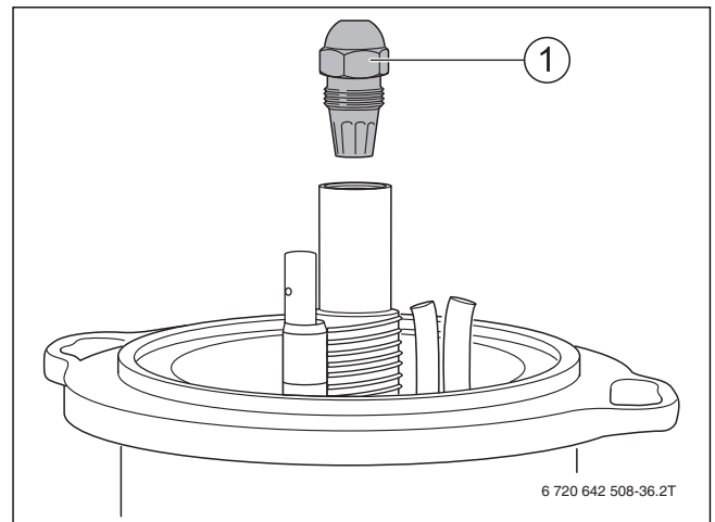
Bild 57 Düse abschrauben
