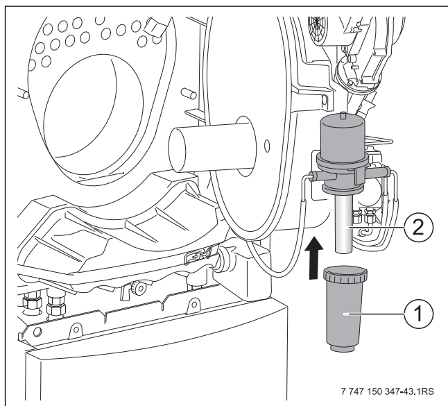
Bild 66 Ölfiltereinsatz wechseln
