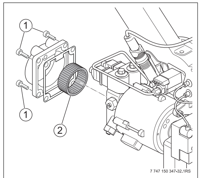
Bild 64 Ölpumpenfilter prüfen
