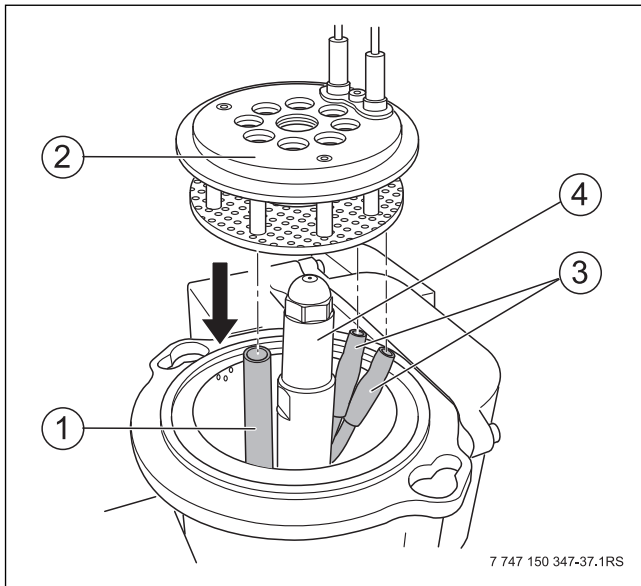
Bild 58 Mischsystem montieren
