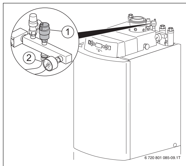
Bild 28 Heizungsanlage befüllen
