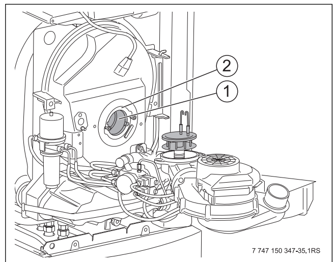
Bild 60 Brennerrohr austauschen
