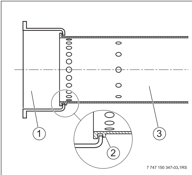
Bild 61 Brennerrohr einsetzen
