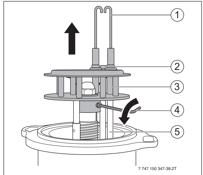
Bild 56 Mischsystem ausbauen
