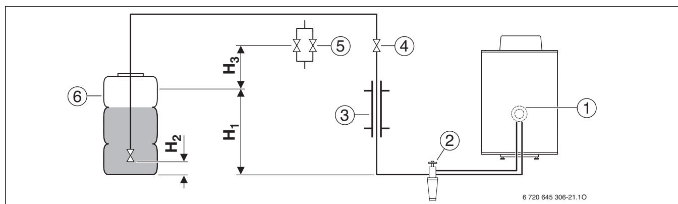
Bild 31 Installationsbeispiel
