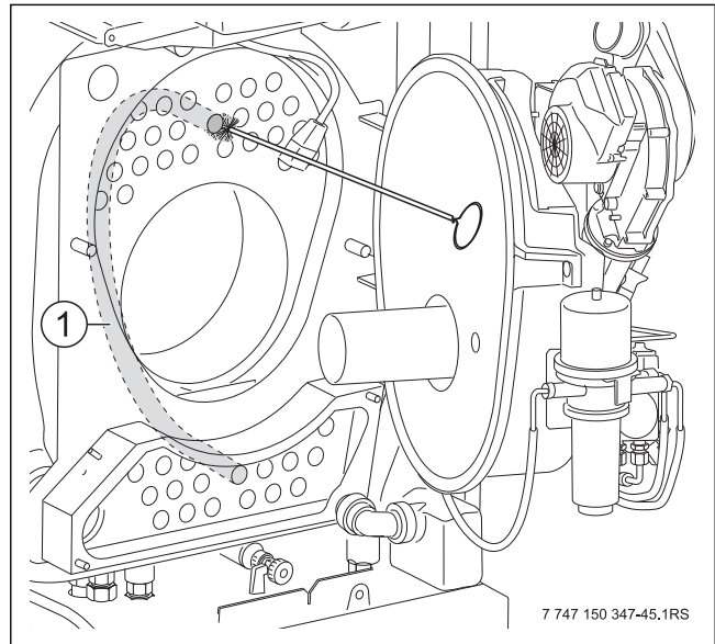
Bild 70 Heizgaszüge reinigen
