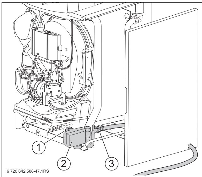
Bild 71 Siphon demontieren
