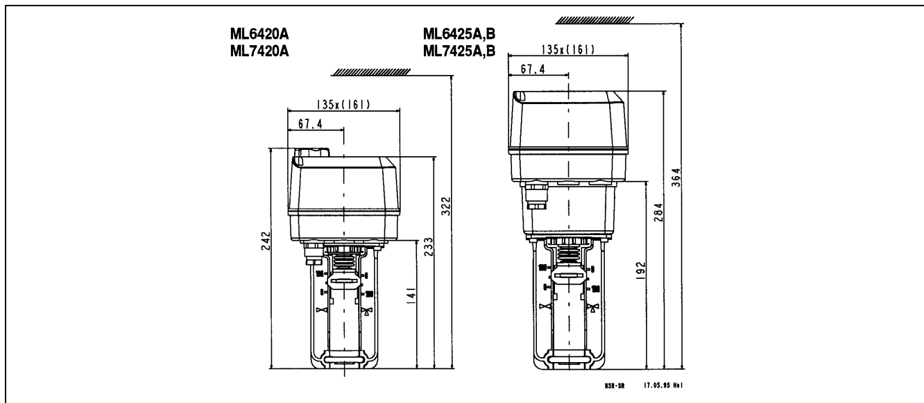
Abb. 3 ML6420A/6425A,B ML7420A/7425A,B
