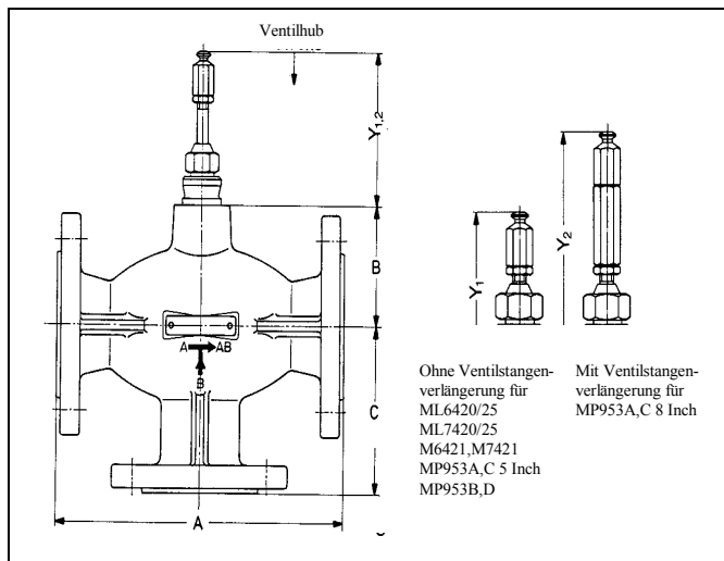
Abb. 1 V5329A,C
