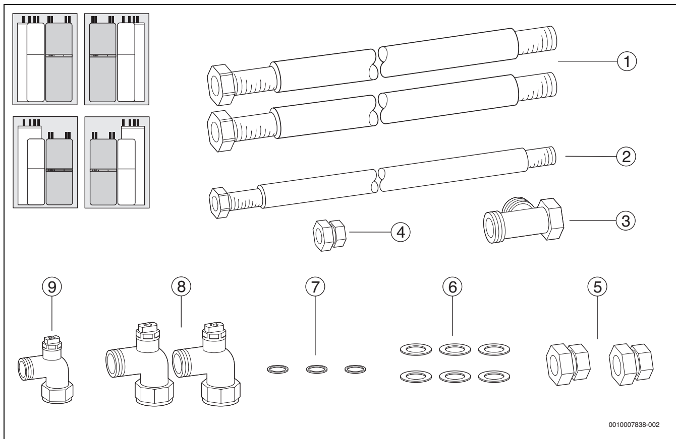
Bild 211 Lieferumfang
