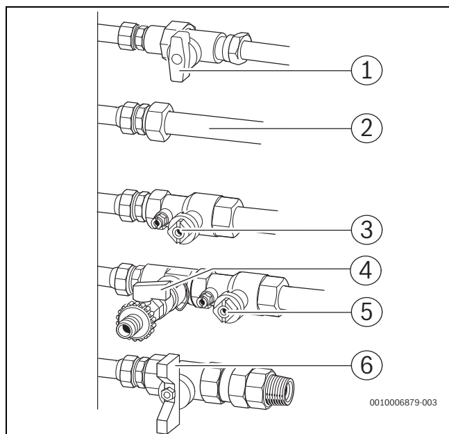
Bild 224 Gas- und wasserseitige Anschlüsse (Beispiel: Anschlusszubehör waagerecht rechts)
