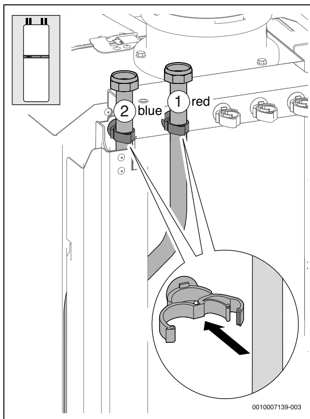
Bild 170
