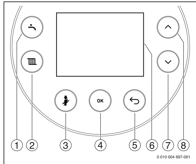
Bild 243 Bedienfeld
