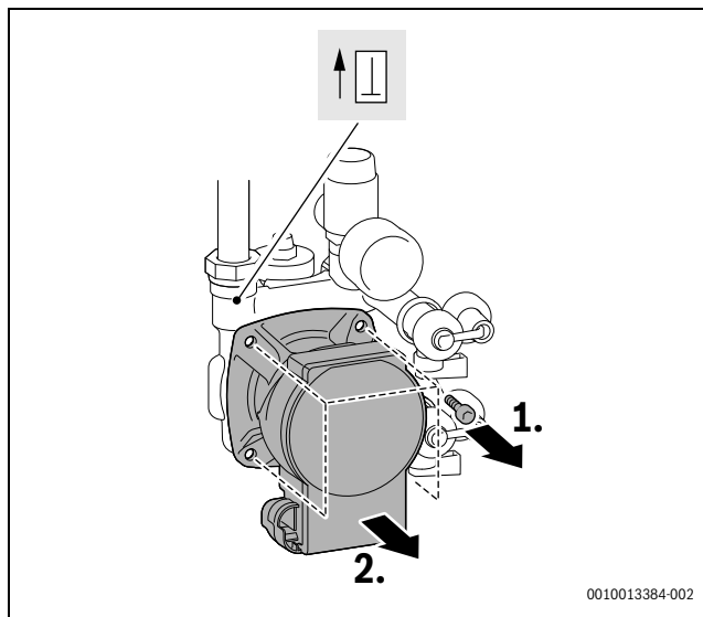
Bild 270 Solarpumpe ausbauen
