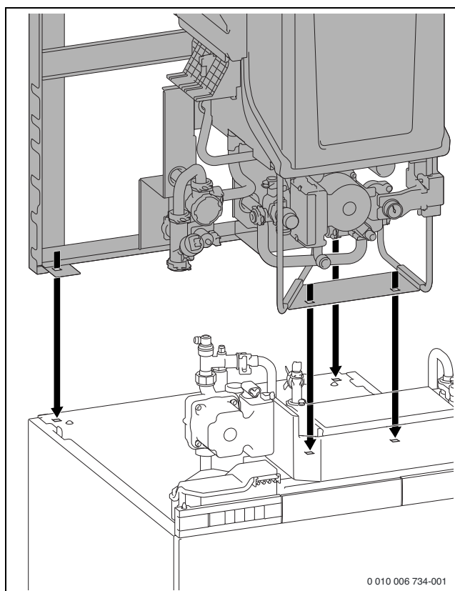
Bild 54 Gerät auf dem Speicher aufsetzen
