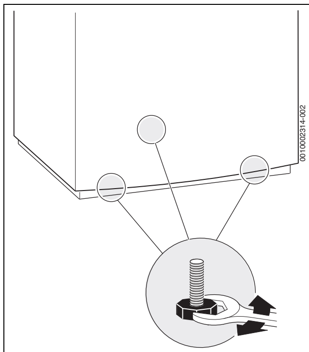
Bild 53 Speicher ausrichten
