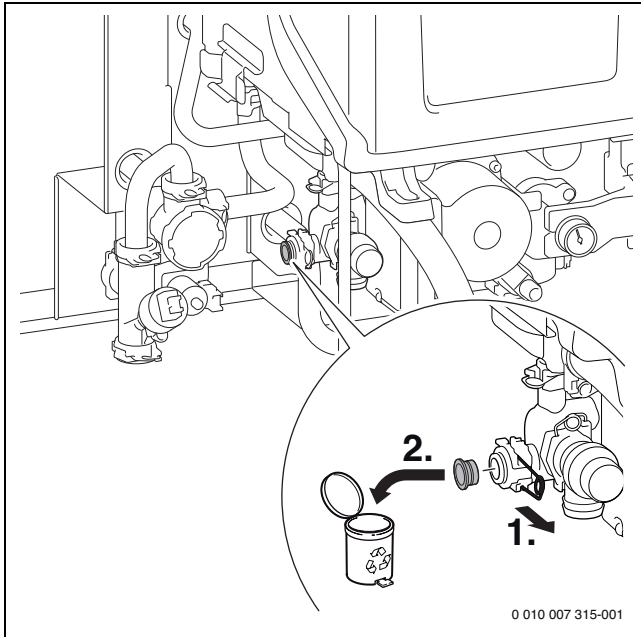
Bild 149 Stopfen entfernen
