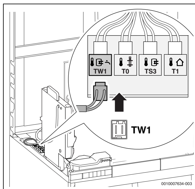
Bild 66 Speichertemperaturfühler anschließen
