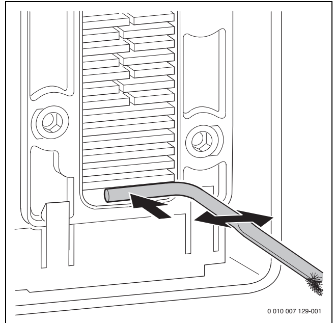
Bild 260 Kondensatwanne reinigen
