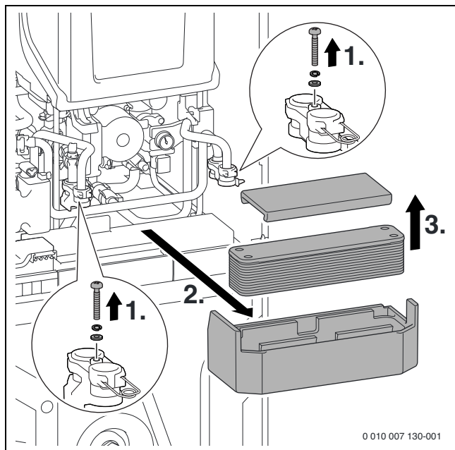
Bild 265 Plattenwärmetauscher ausbauen
