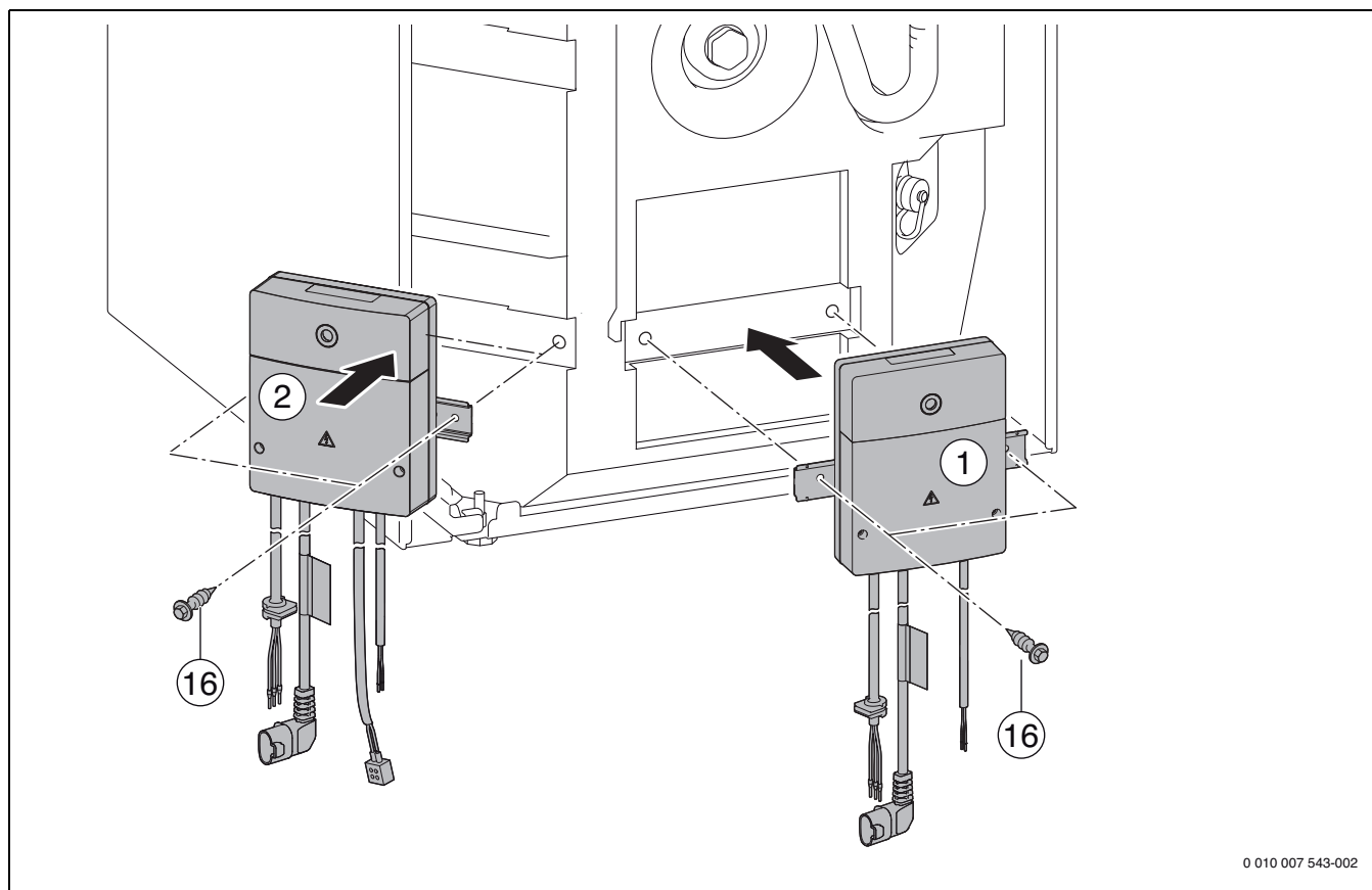
Bild 138 GC9000iWM../100-Geräte
