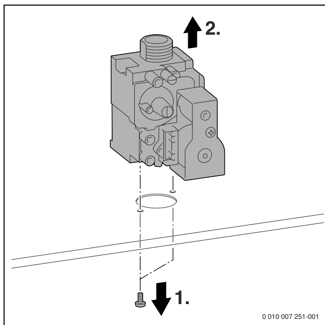
Bild 269 Gasarmatur ausbauen
