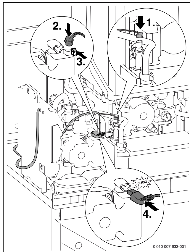
Bild 65 Speicherladepumpe und Warmwasser-Temperaturfühler anschließen
