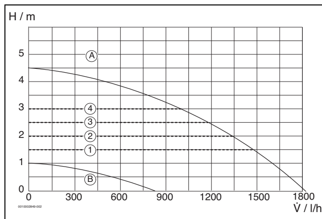
Bild 275 Pumpenkennfelder und Pumpenkennlinien
