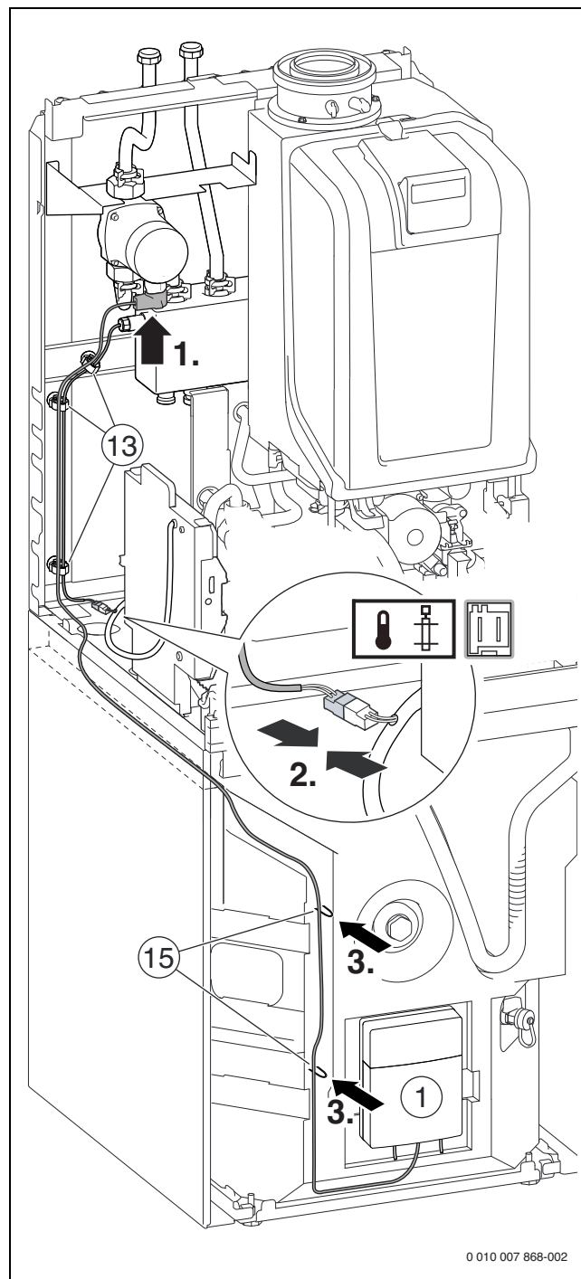
Bild 112 GC9000iWM../100-Geräte: Anschluss Heizungspumpe ungemischter Heizkreis und Hydraulische Weiche
