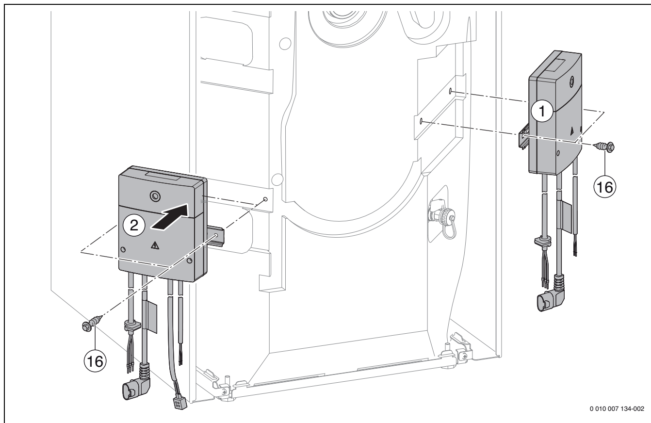
Bild 137 GC9000iWM../150-Geräte
