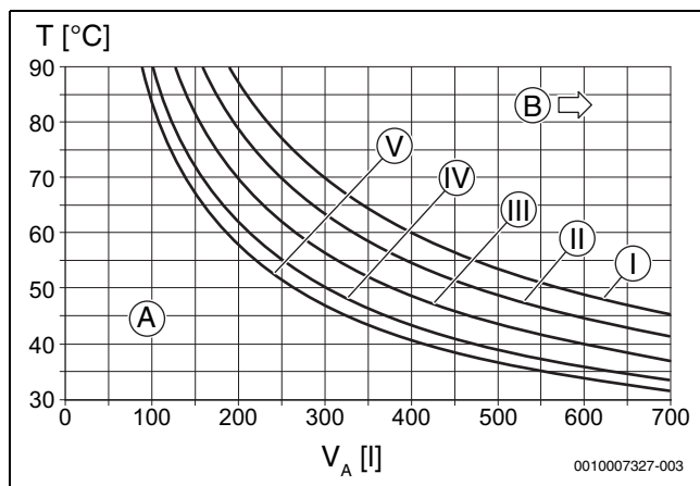
Bild 46 Kennlinien des Ausdehnungsgefäßes 17 l
