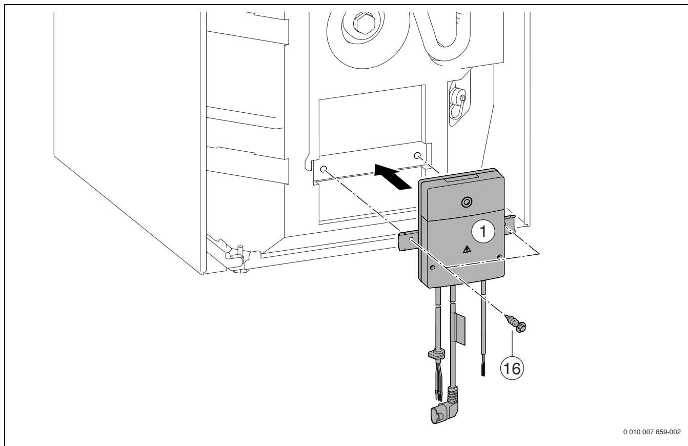
Bild 110 GC9000iWM../100-Geräte
