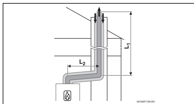
Bild 27 Konzentrische Luft-Abgas-Führung nach C 33x im Schacht
