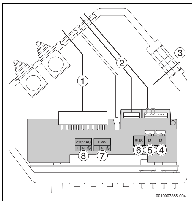
Bild 228 Anschlussbox
