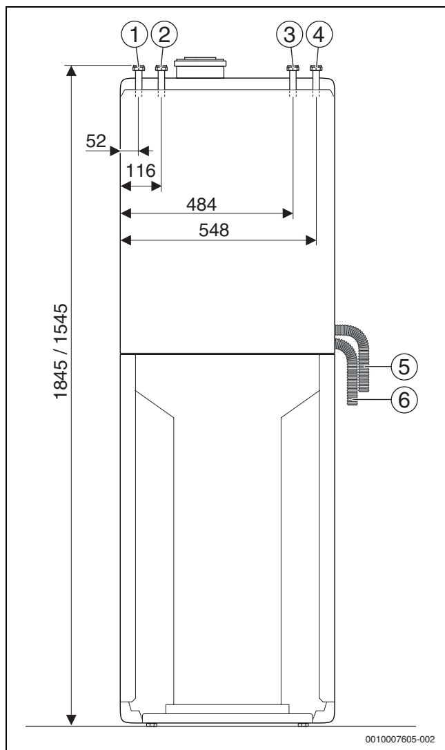
Bild 15 Anschlussmaße des Zubehörs CS 15 - Anschluss-Set solare Heizungsunterstützung (Maße in mm)
