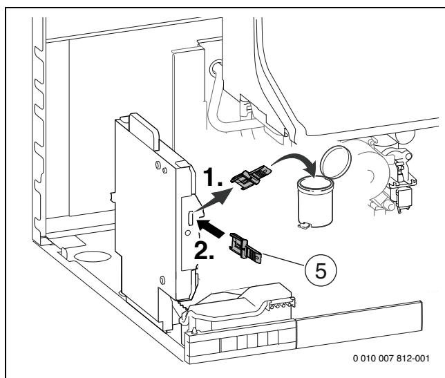
Bild 152 Kodierstecker tauschen
