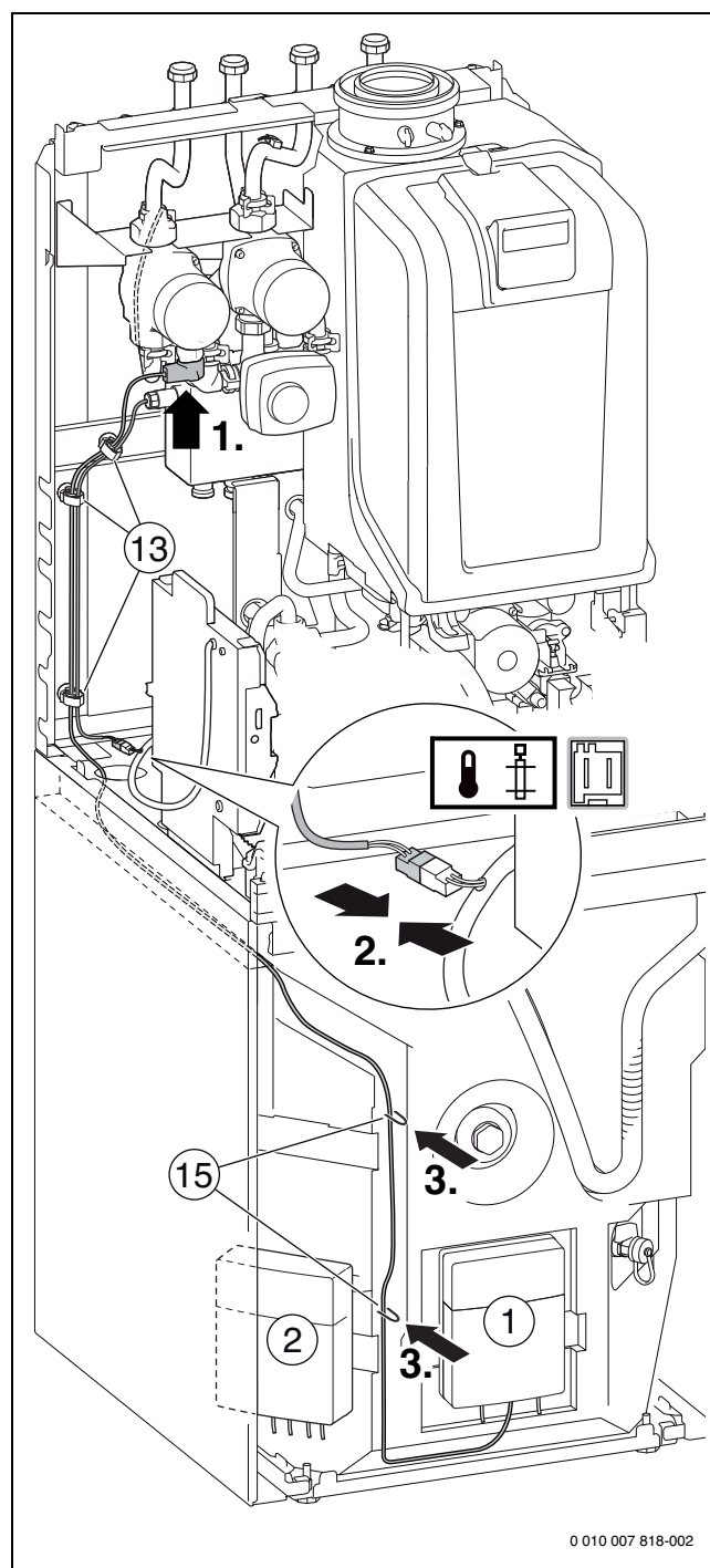
Bild 140 GC9000iWM../100-Geräte: Anschluss Heizungspumpe ungemischter Heizkreis und Hydraulische Weiche
