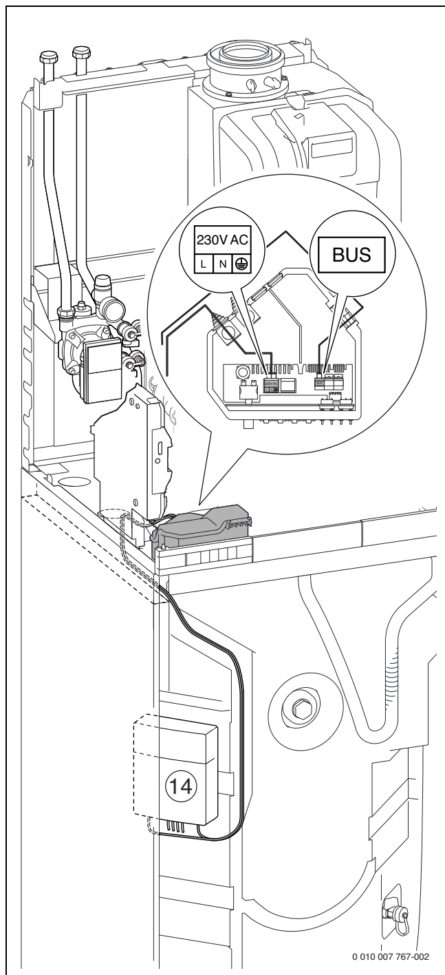
Bild 178 GC9000iWM../150-Geräte
