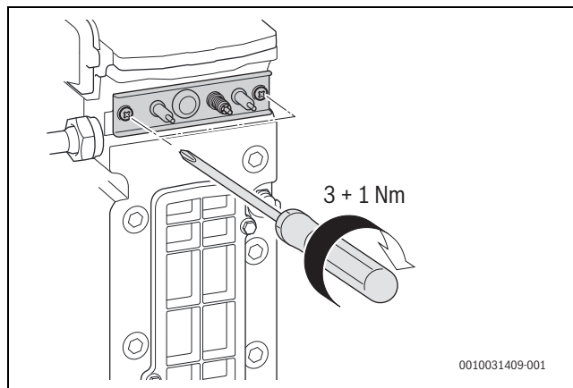
Bild 252 Elektroden-Set wieder einbauen
