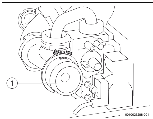
Bild 247 Gas-Luft-Verhältnis einstellen
