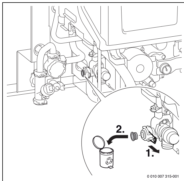
Bild 115 Stopfen entfernen
