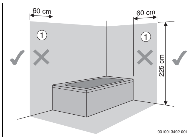
Bild 225 Schutzbereiche
