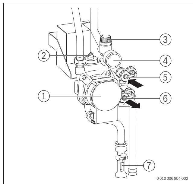
Bild 236 Übersicht Solargruppe
