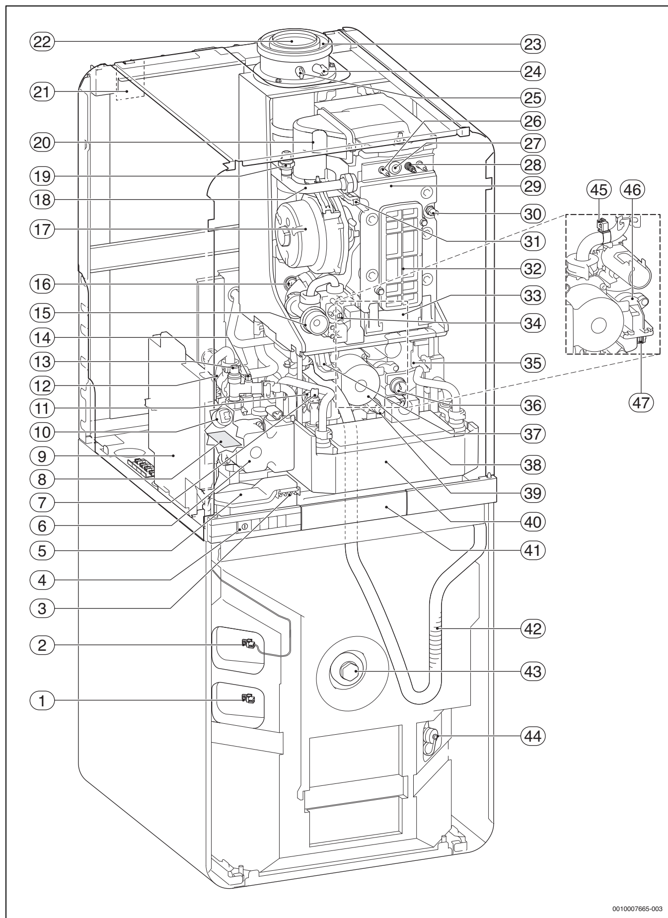
Bild 19 GC9000iWM.../100.-Geräte
