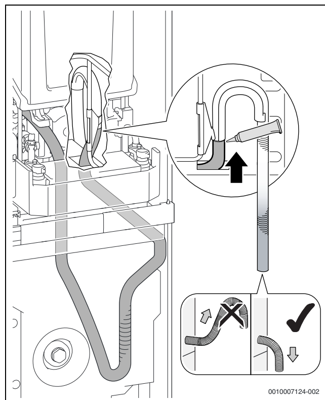
Bild 58 Siphonschlauch am Endstück einstecken
