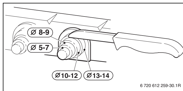
Bild 145 Zugentlastung Kabel Mischermotor anpassen
