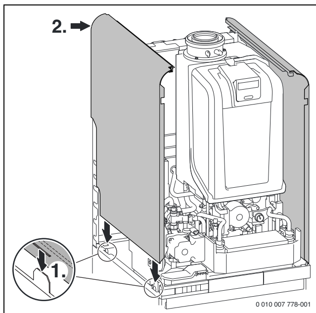
Bild 238 Rechte und linke Verkleidung montieren
