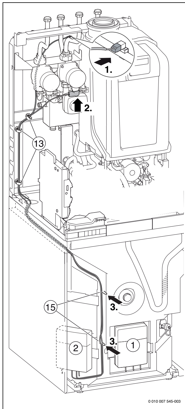
Bild 142 GC9000iWM ../100-Geräte: Anschluss Heizungspumpe gemischter Heizkreis und Temperaturfühler
