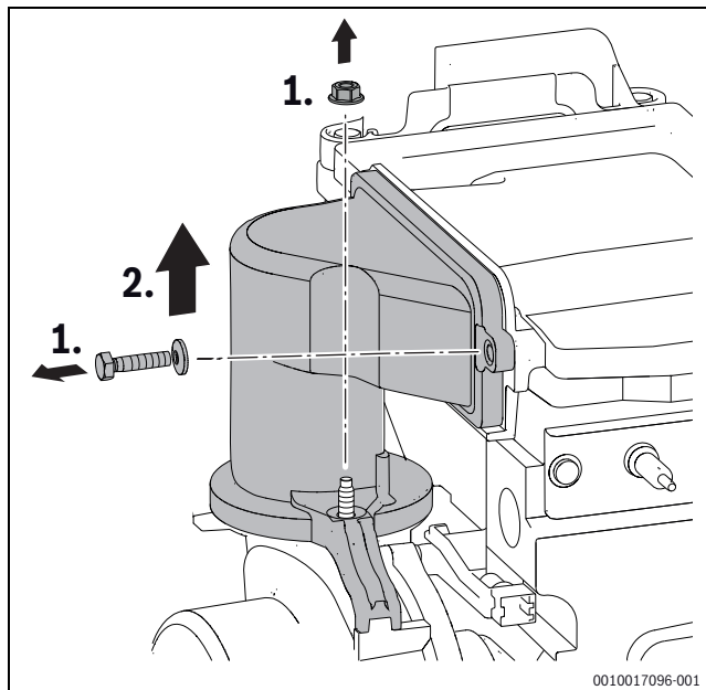
Bild 263 Mischeinrichtung ausbauen
