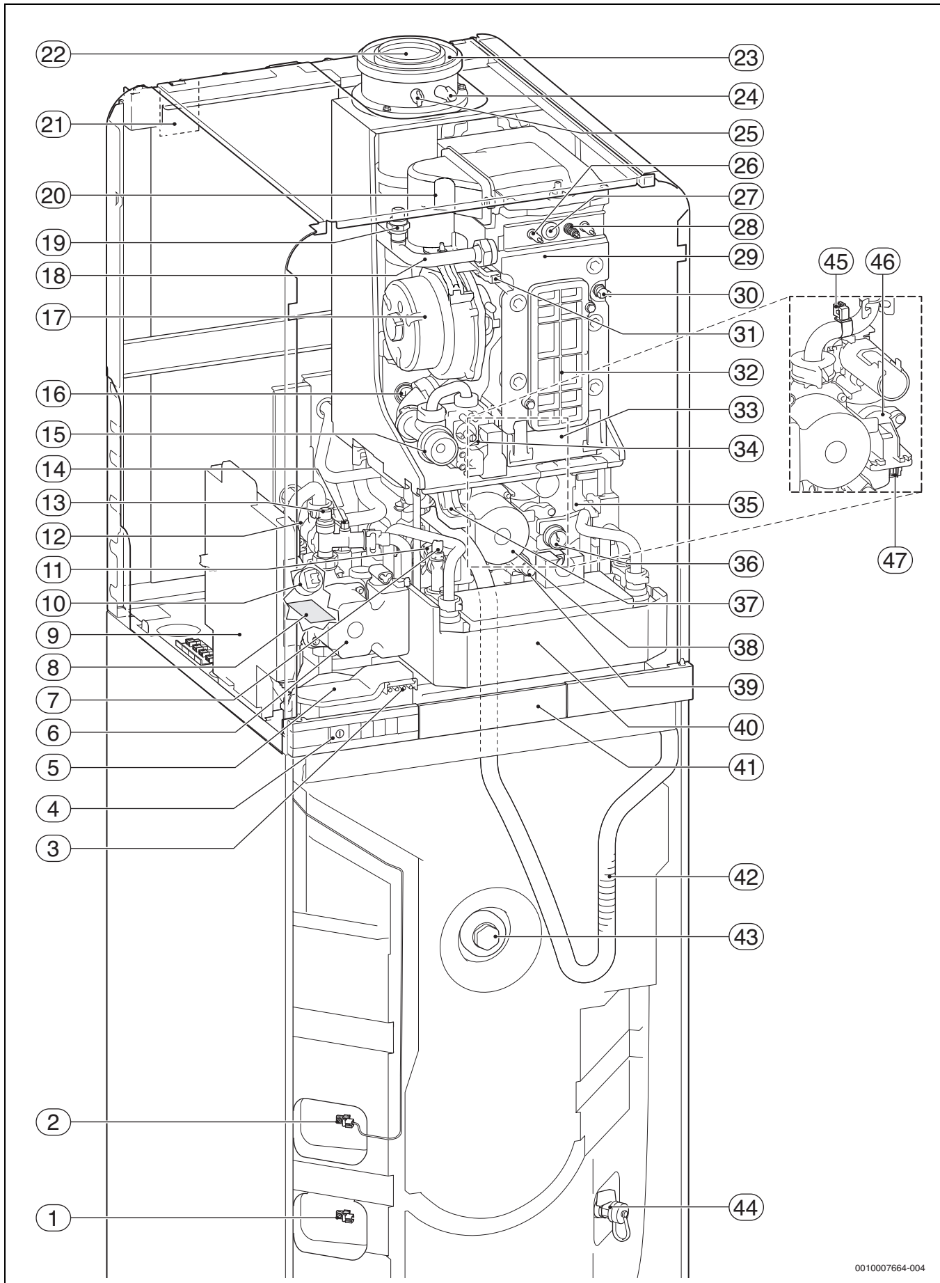
Bild 18 GC9000iWM.../150..-Geräte
