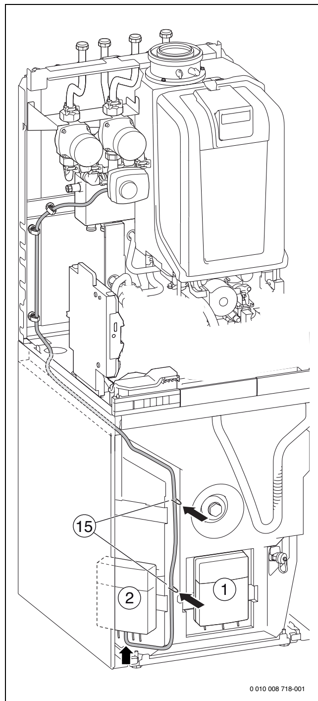
Bild 144 GC9000iWM ../100-Geräte: Anschluss Mischermotor
