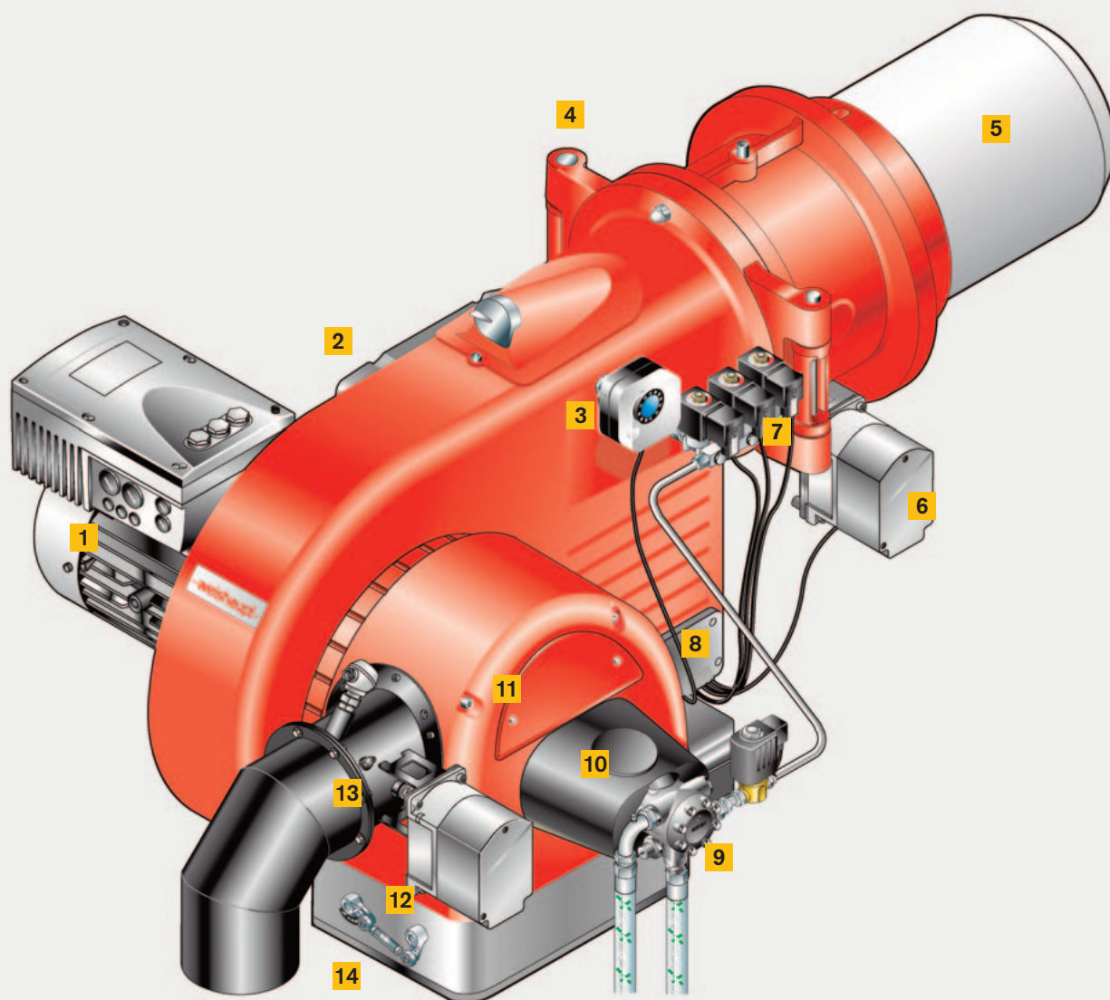
WM-GL20 Ausföhrung ZM-T-4LN
